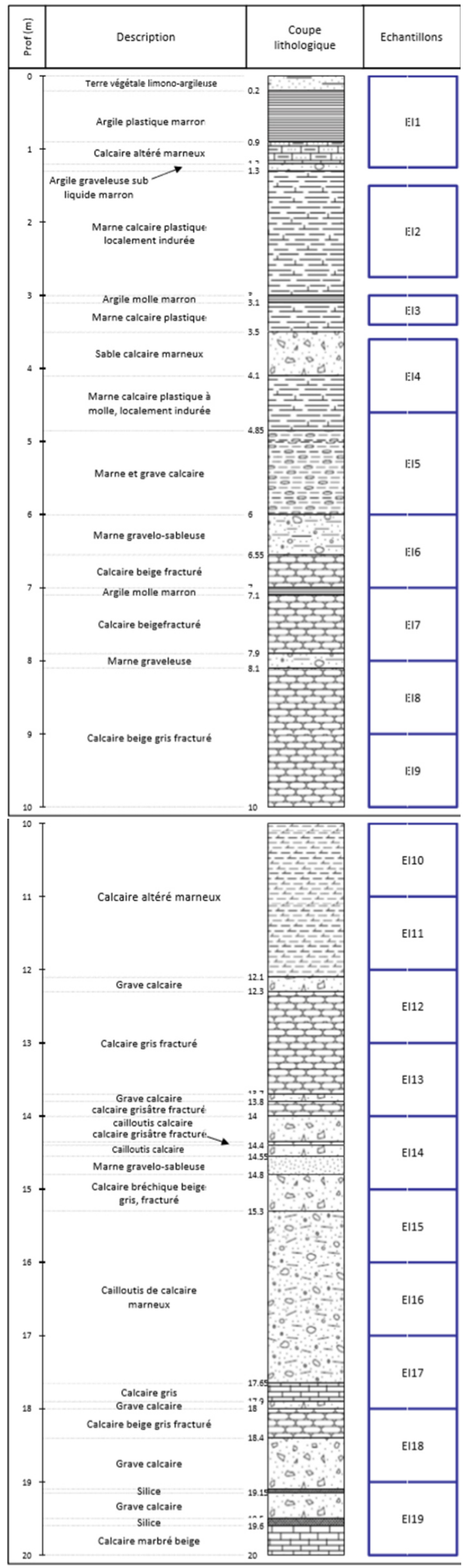
Figure 11- 33 Coupe lithologique du sondage carotté SC2 au lieu-dit « les Hôtels ».
