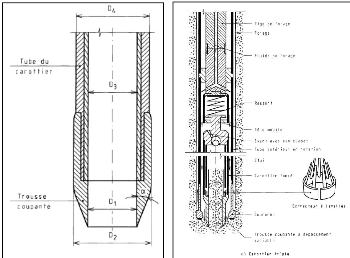
a. Carottier de type poinçonneur b. Carottier triple Figure 10- 3 Schémas des carottiers utilisés pour les sondages carottés SC (Stemmans et al., 2009)
