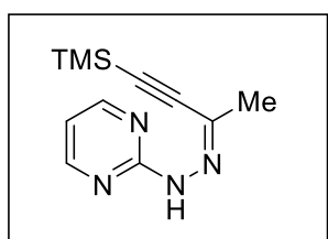
(Z)-2-(2-(4-(Trimethylsilyl)but-3-yn-2-ylidene)hydrazinyl)pyrimidine (93i)
