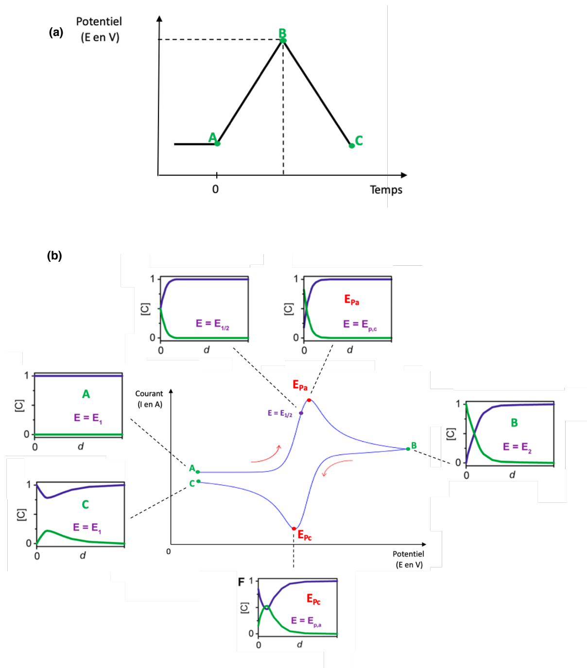
Figure 2 : Voltammétrie cyclique d'un système réversible : (a) Potentiel appliqué en fonction du temps pour une expérience de voltampérométrie cyclique, les potentiels initial, intermédiaire et final étant représentés (A, B et C, respectivement) ; (b) Allure du voltamogramme cyclique réversible résultant avec I_{Pa} , le courant anodique ; I_{Pc} , courant cathodique ; E_{Pa} , potentiel d'oxydation anodique ; E_{Pc} , potentiel de réduction cathodique et E_{1/2} , le potentiel à mi-hauteur du pic cathodique. Représentation des profils de concentrations pour l'oxydant Fc^+ (en bleu) et le réducteur Fc (en vert) aux points caractéristiques du voltamogramme.
