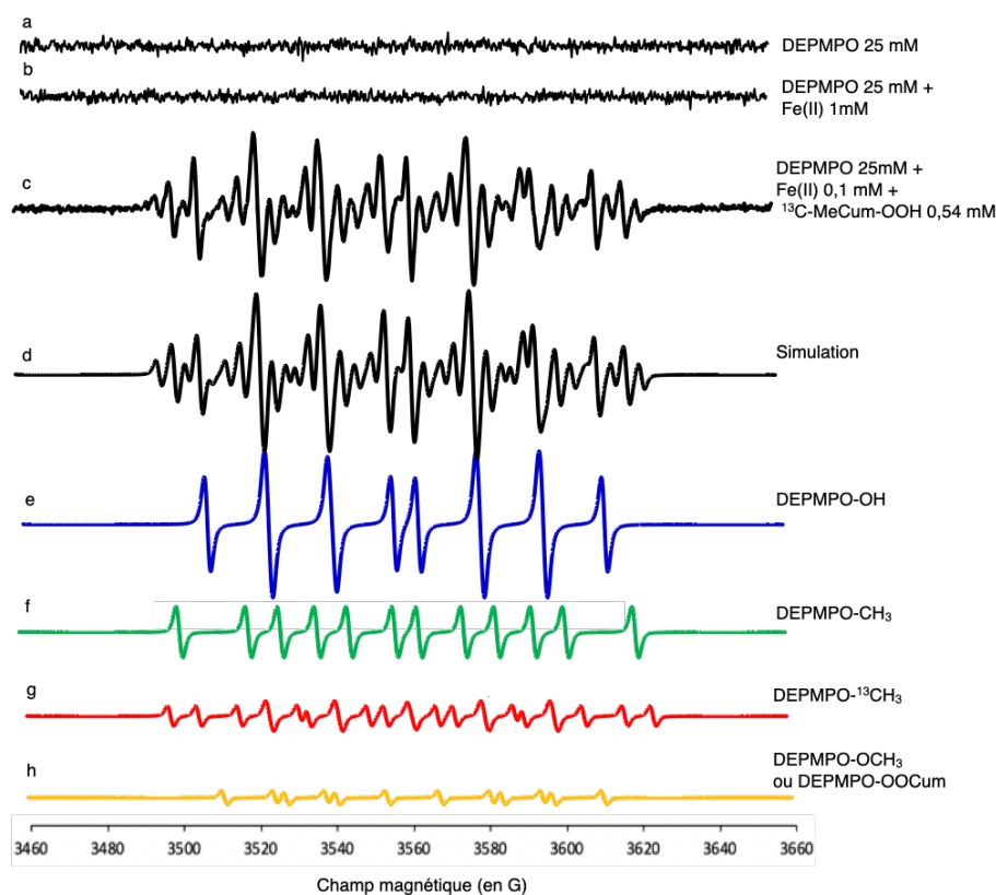
Figure 48 : Spectres de RPE concernant le ^{13}\text{C-MeCum-OOH} (a) contrôle-DEPMPPO 25 mM seul ; (b) contrôle-DEPMPPO 25 mM/Fe(II) 1 mM ; (c) spectre expérimental pour le ^{13}\text{C-MeCum-OOH} 0,54 mM/Fe(II) 0,1 mM/DEPMPPO 25 mM ; (d) simulation avec Easyspin/Matlab et (e); DEPMPPO-OH (ca. 45 %) ; DEPMPPO-CH 3 (ca. 28 %) ; DEPMPPO- ^{13}\text{CH}_3 (ca. 23 %) et DEPMPPO-OCH 3 ou DEPMPPO-OOCum (< 5 %).
