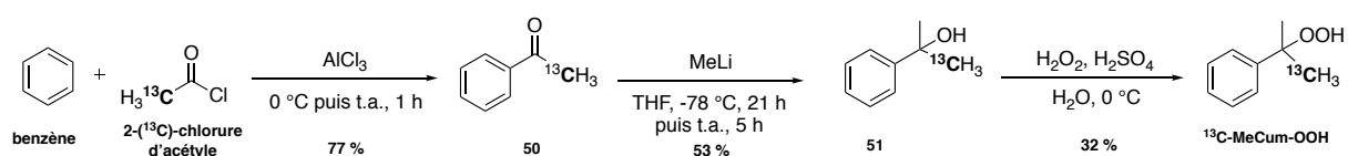
Figure 45 : Synthèse du 13 C-MeCum-OOH.
