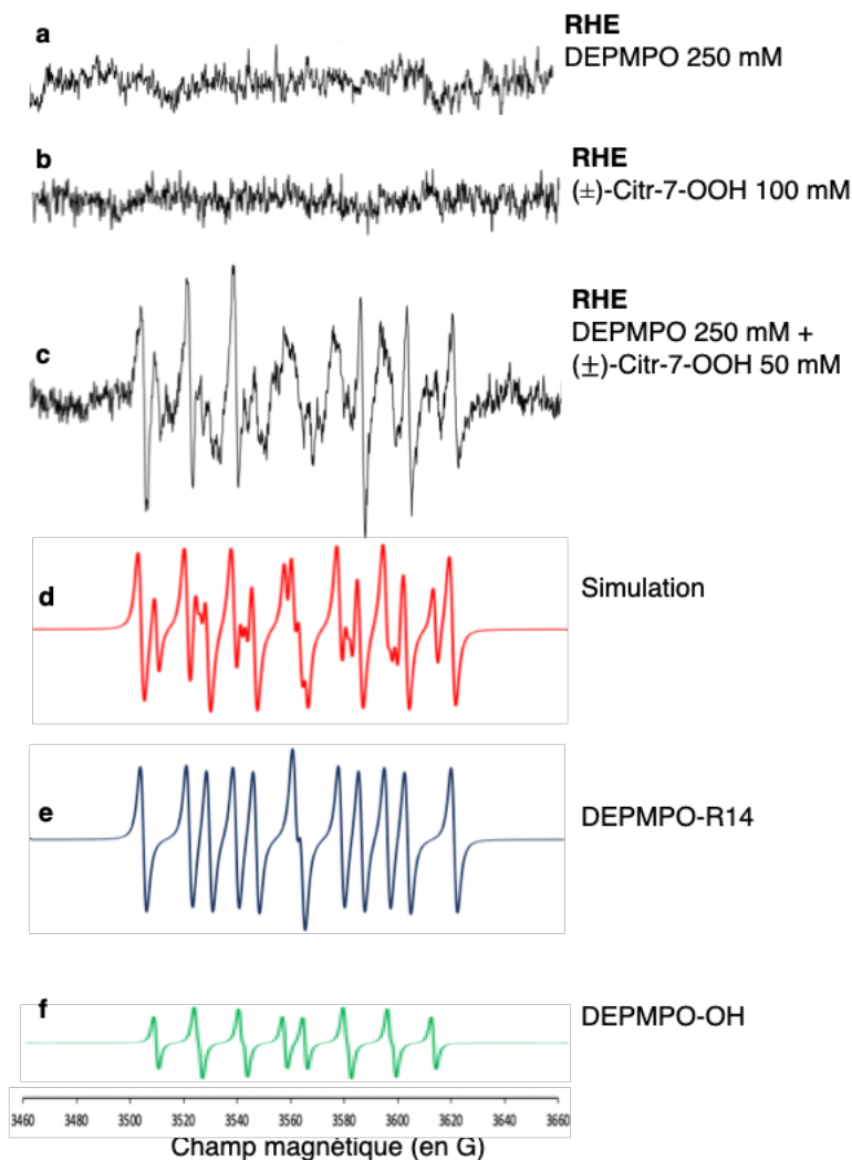
Figure 42 : Étude RPE sur RHE- (\pm) -Citr-7-OOH (a) contrôle RHE-DEPMPO 250 mM ; (b) contrôle RHE- (\pm) -Citr-7-OOH (100 mM) (c) spectre RHE sur RHE après incubation de DEPMPO 250 mM suivie d'une addition (\pm) -Citr-7-OOH 50 mM ; (d) simulation de (c) et sa déconvolution en DEPMPO-R14 (e) (ca. 77 %) et DEPMPO-OH (f) (ca. 23 %).
