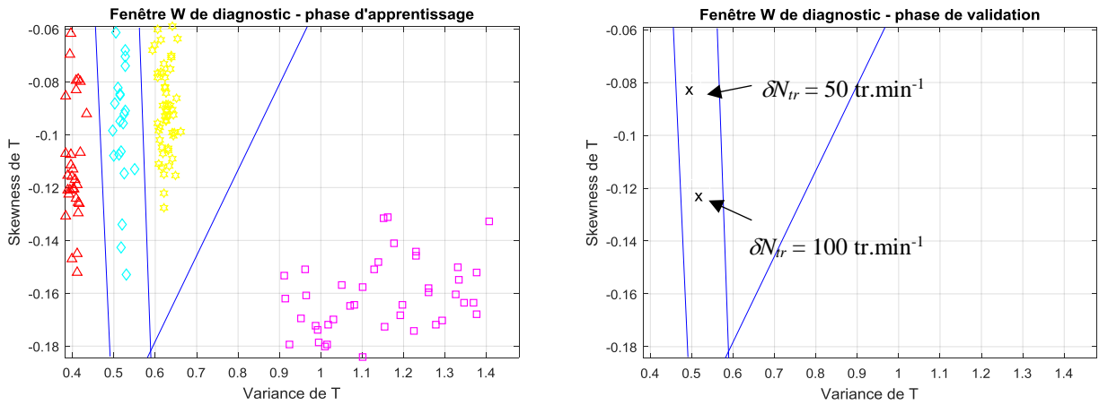
Figure IV.A7. Localisation des défauts \delta N_{tr} à t = 0\text{s} dans la fenêtre W = [350\text{s} : 650\text{s}] .
