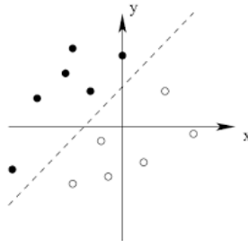
Figure IV.4. Exemple de séparateur linéaire.
