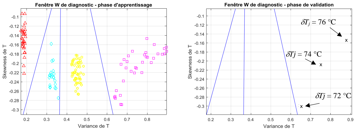
Figure IV.A6. Localisation des défauts \delta T_j à t = 600\text{s} dans la fenêtre W = [650\text{s} : 950\text{s}] .
