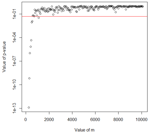
Figure 57 : p - value pour chaque KS-test effectué sur des échantillons de données de différentes tailles m récoltés sur le lien 1
