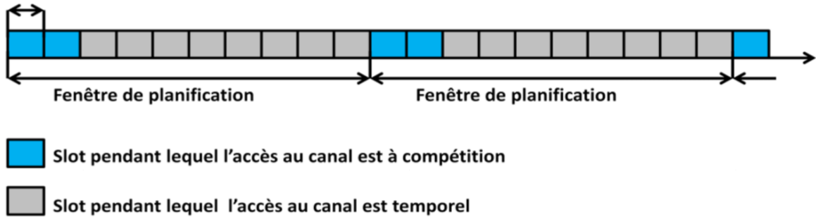
Figure 19 : Division du temps en fenêtres de planification composées de 10 slots ( N = 10 ) dont 2 sont réservés à l'accès à compétition au canal ( N_c = 2 ) et 8 à l'accès temporel au canal ( N_p = 8 )
