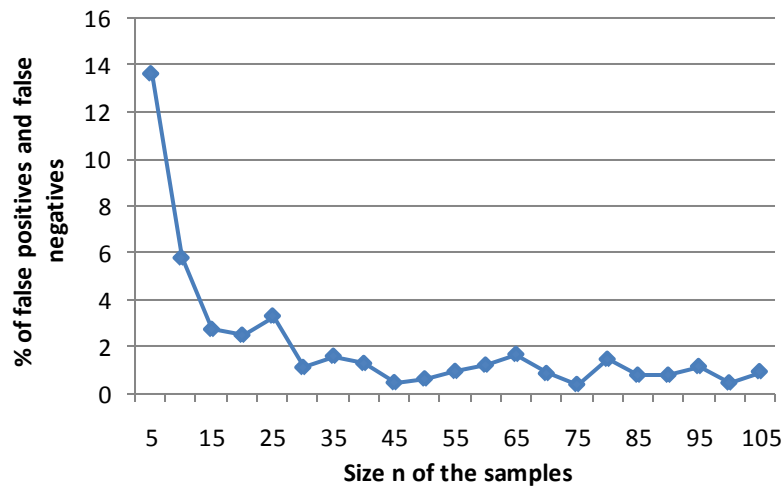
Figure 62 : Pourcentage de faux négatifs et de faux positifs lorsque les échantillons sont de taille n et que l'écart-type de la loi normale tronquée en 0 et en 1 générant les échantillons est de 0.1 ( \sigma_{ij}^o = 0.1 ).
