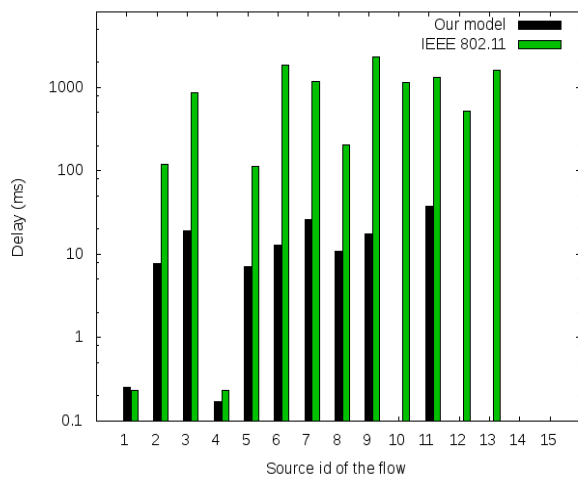
Figure 43 : Délai des flux dans le réseau mesh à topologie maillée
