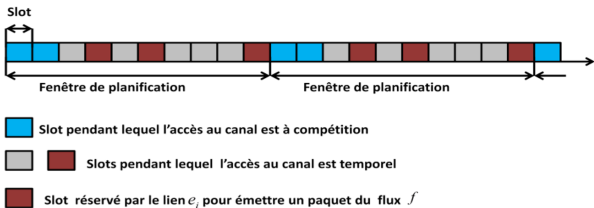
Figure 22 : Le nœud e_i a réservé trois slots pour le flux f par fenêtre de planification
