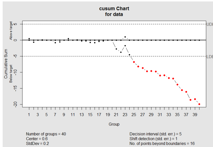
Figure 60: Carte de contrôle établie par la méthode CUSUM sur un échantillon de 40 données
