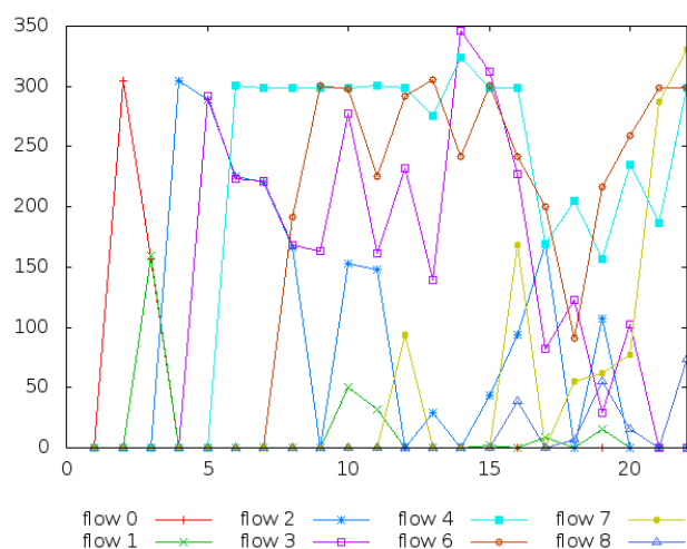
Figure 35 : Débit des flux en kbit/s dans le temps (seconde) avec le modèle original sur la topologie chaînée
