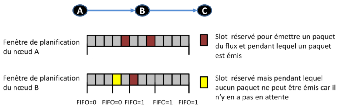
Figure 25 : Illustration du phénomène de slots perdus , lorsqu'un nœud ne peut émettre de paquet lors d'un slot réservé car il n'en possède aucun en attente
