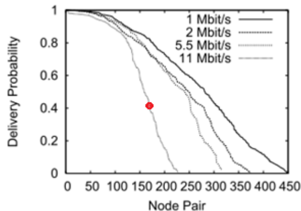
Figure 52 : Distribution de la probabilité de perte de paquets. Chaque point correspond à une paire émetteur/récepteur à un débit particulier. Seuls les paires émetteur/récepteur qui ont envoyé au moins un paquet avec succès pendant l'expérience, sont représentées sur la figure (Aguayo, et al. 2004).
