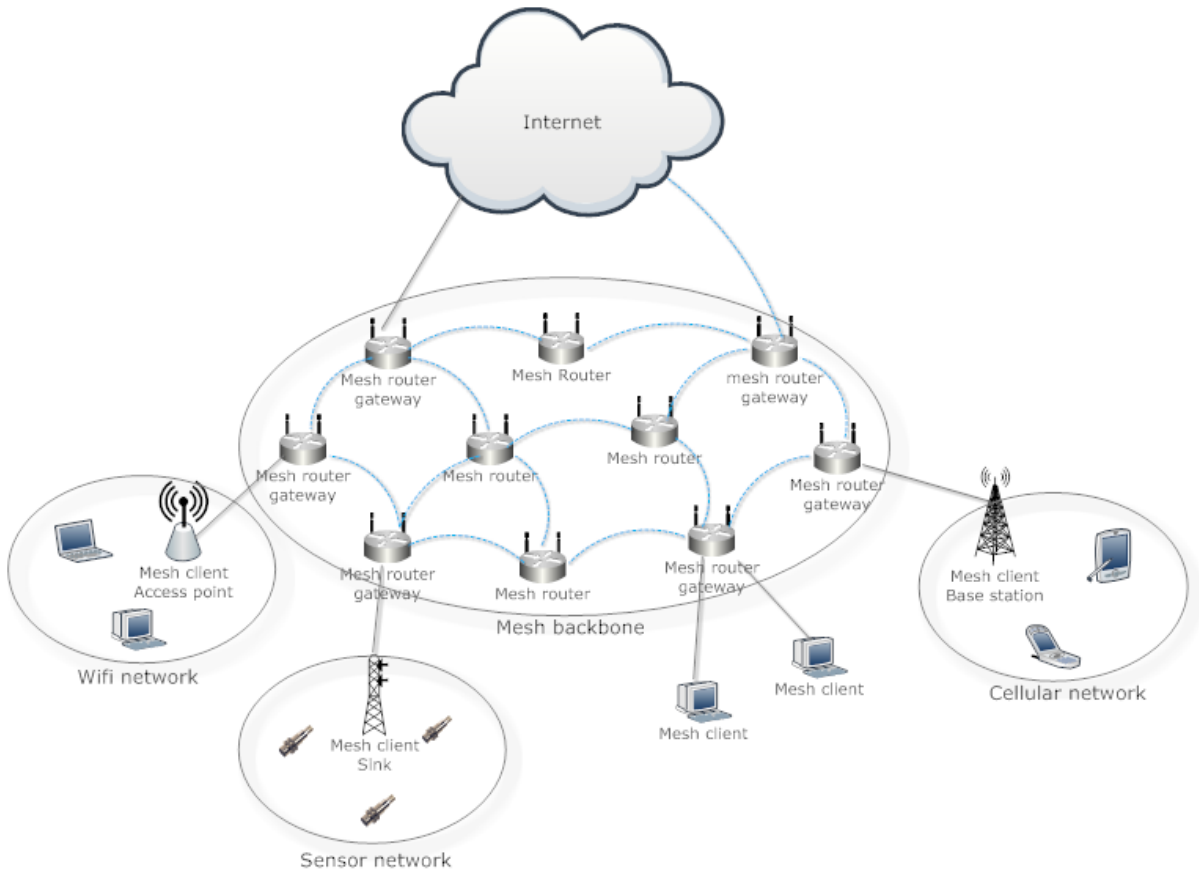
Figure 3: Exemple d'un réseau
