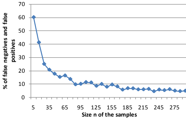
Figure 63 : Pourcentage de faux négatifs et de faux positifs lorsque les échantillons sont de taille n et que l'écart-type de la loi normale tronquée en 0 et en 1 générant les échantillons est de 0.5 ( \sigma_{ij}^o = 0.5 ).
