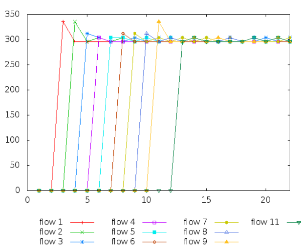
Figure 38 : Débit des flux en kbit/s dans le temps (seconde) avec notre modèle sur un réseau à topologie maillée.
