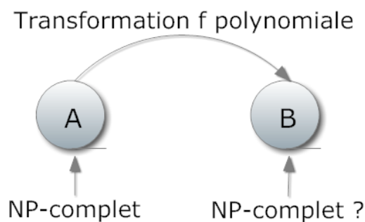
Figure 26 : Le problème A qui est NP-complet est transformable en un problème B via une fonction polynomiale f . Si B est également NP alors le problème B est NP-complet.
