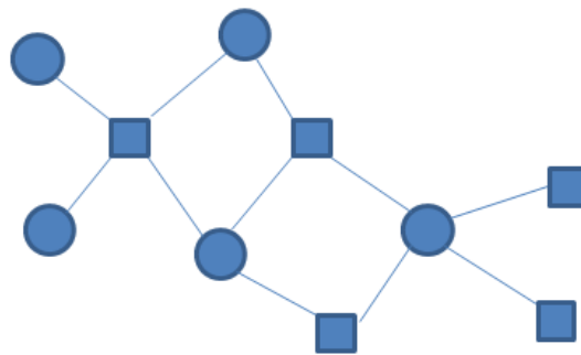
Figure 27 : Graphe biparti planaire extérieur. Chaque arête a un sommet carré et un sommet rond ; le graphe est donc bien biparti.
