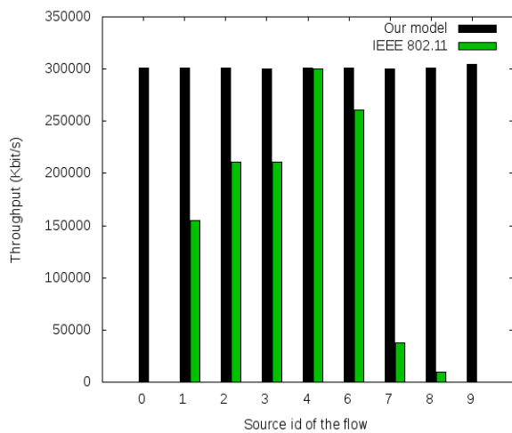
Figure 40 : Comparaison du débit des flux du réseau à topologie chaînée
