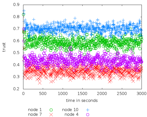
Figure 81 : Confiance des nœuds dans un réseau mesh à topologie en croix avec la solution de référence lorsque p=0.5
