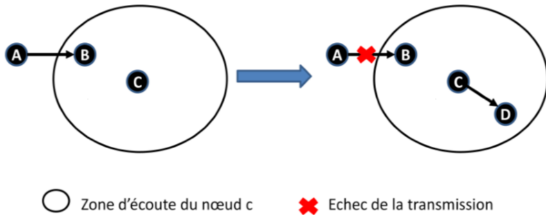
Figure 11 : C est un nœud caché de la communication entre A et B
