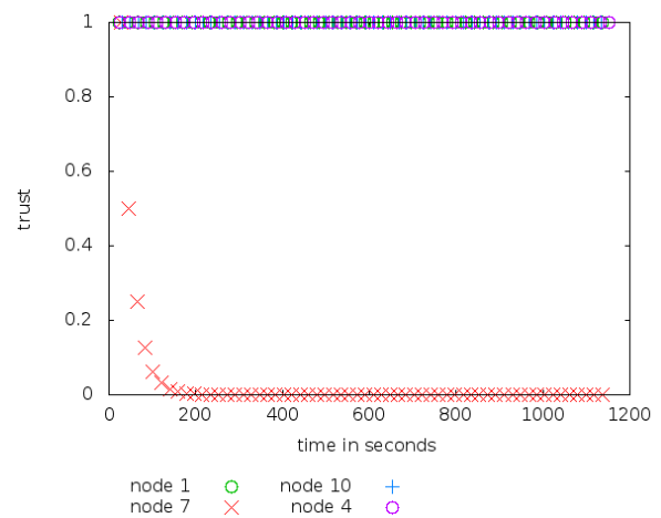
Figure 80 : Confiance des nœuds dans un réseau mesh à topologie en croix avec notre solution lorsque p=1
