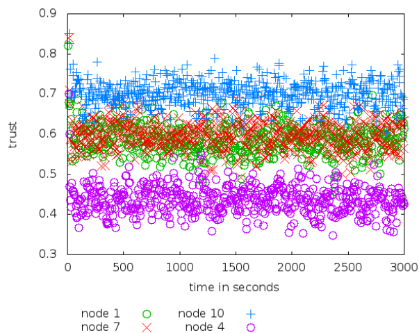
Figure 83 : Confiance des nœuds dans un réseau mesh à topologie en croix avec la solution de référence lorsque p=0.2
