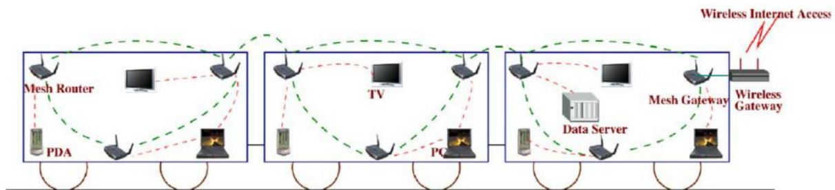
Figure 7 : Un réseau mesh sans fil déployé dans un train (Akyildiz, Wang et Wang 2005)
