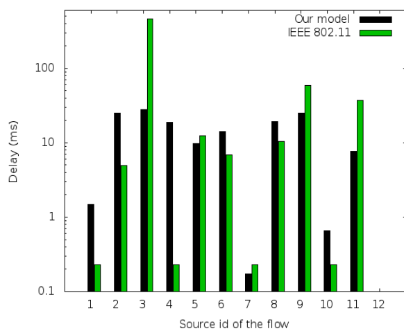
Figure 44 : Délai des flux dans le réseau mesh à topologie en croix
