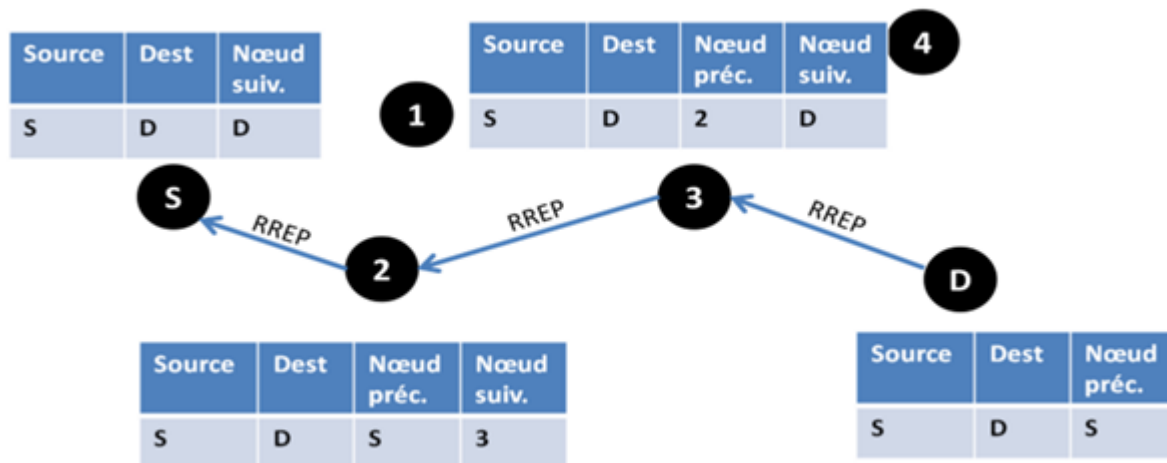
Figure 5 : envoi d'un RREP par la destination D le long du chemin emprunté par le RREQ
