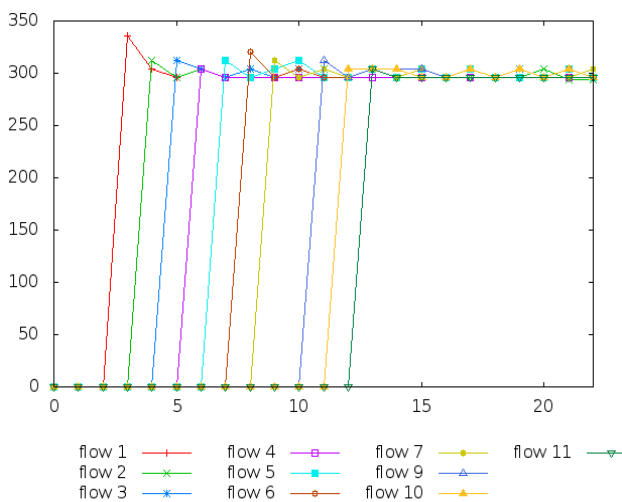
Figure 36 : Débit des flux en kbit/s dans le temps (seconde) avec notre modèle sur la topologie en croix.
