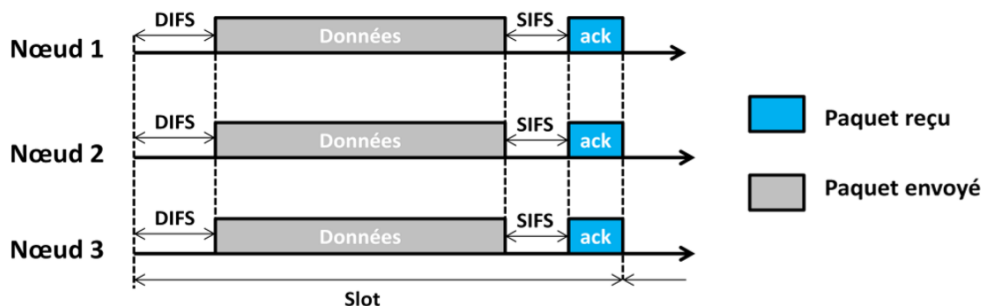
Figure 21 : Trois nœuds envoient un paquet de données sur un même slot
