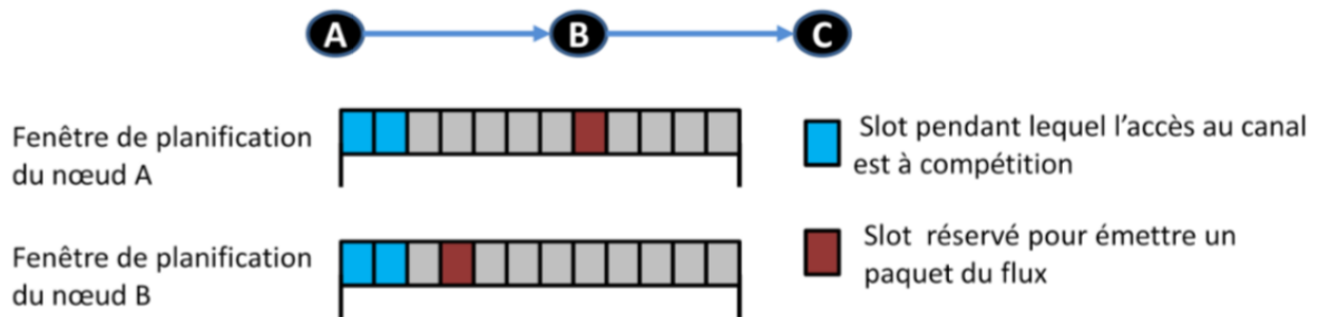
Figure 24 : Le nœud B émet le paquet en provenance de A au cours de la fenêtre de planification suivant celle où il a reçu le paquet.
