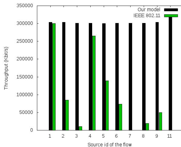
Figure 42 : Comparaison du débit des flux pour la topologie maillée
