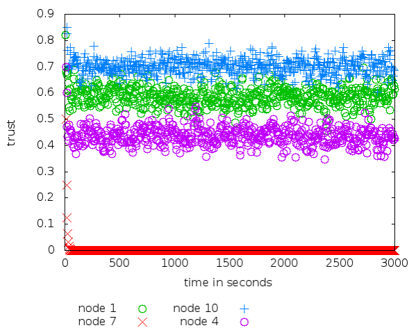
Figure 79 : Confiance des nœuds dans un réseau mesh à topologie en croix avec la solution de référence lorsque p=1
