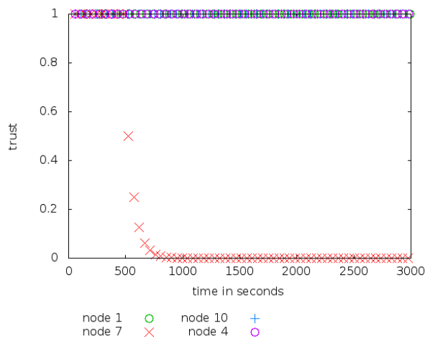
Figure 84 : Confiance des nœuds dans un réseau mesh à topologie en croix avec notre solution lorsque p=0.2
