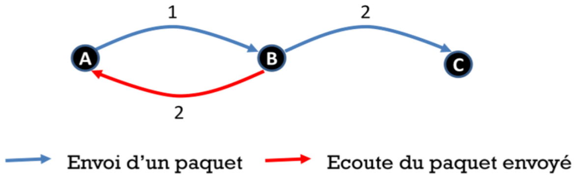
Figure 47 : Illustration de Watchdog : A envoie un paquet à B et vérifie que B le fait suivre à C en écoutant les paquets que B envoie.
