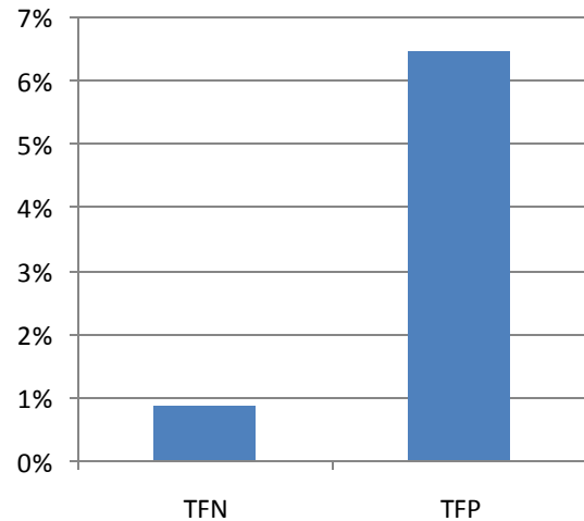
Figure 68 : Taux de faux négatifs et faux positifs lorsque \sigma_{ij}^o=0.5 et n = 250
