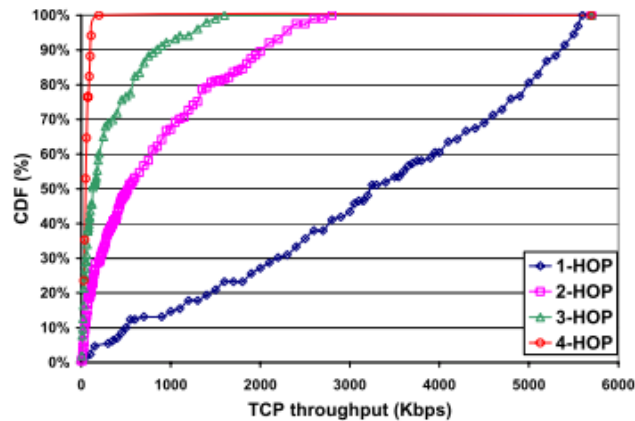
Figure 1 : Fonction de répartition du débit de flux TCP selon la distance entre leur nœud source et la destination, sachant qu'une seule session TCP est active à la fois. Chaque flux est émis à 5Mbit/s (Das, Koutsonikolas et Hu 2008).
