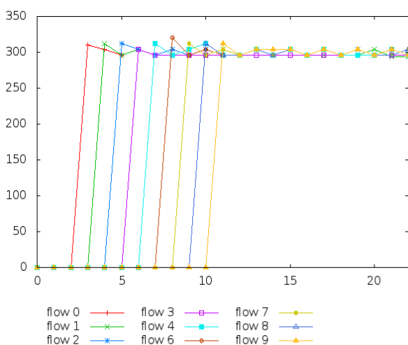
Figure 34: Débit des flux en kbit/s dans le temps (seconde) avec notre modèle sur la topologie chaînée
