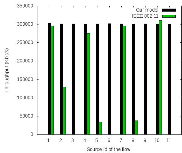
Figure 41 : Comparaison du débit des flux pour la topologie en croix
