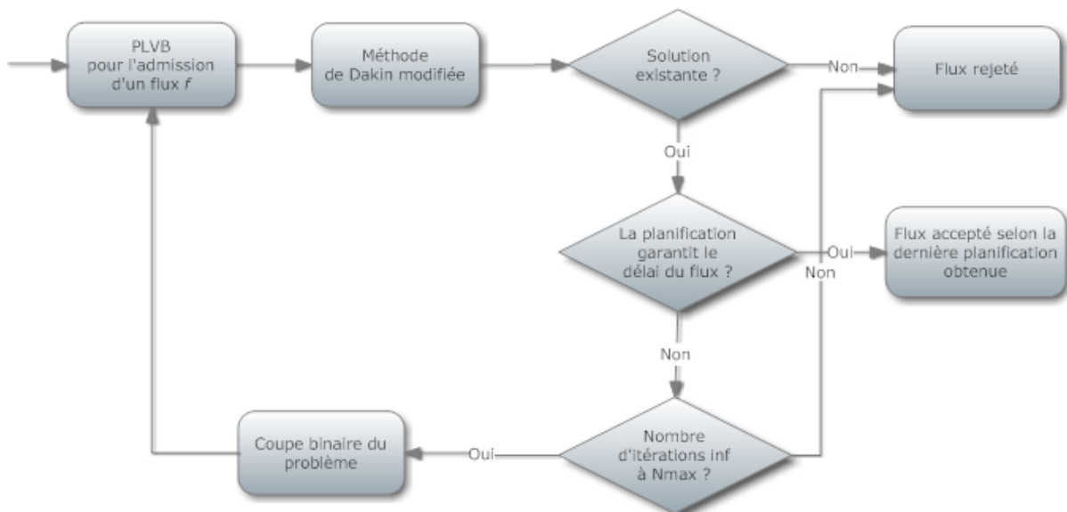
Figure 30 : Approche itérative de l'algorithme d'admission et de planification d'un flux
