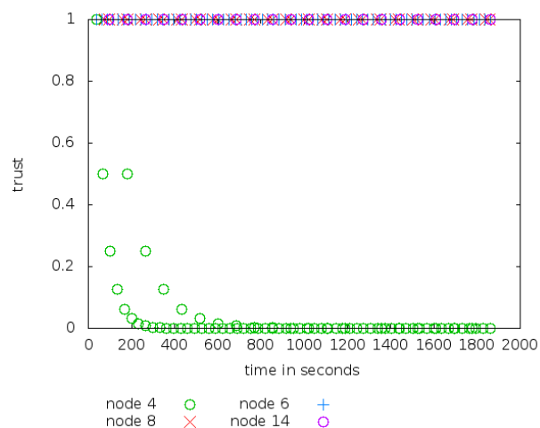
Figure 86 : Confiance des nœuds dans un réseau mesh à topologie maillée avec notre solution lorsque p=0.2
