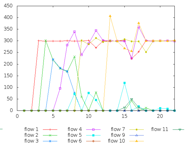
Figure 37: Débit des flux en kbit/s dans le temps (seconde) avec le modèle originel sur la topologie en croix.
