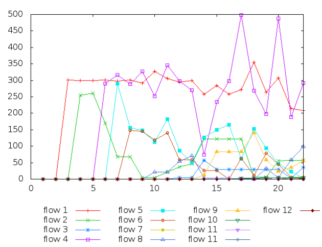
Figure 39 : Débit des flux en kbit/s dans le temps (seconde) avec le modèle originel sur un réseau à topologie maillée.
