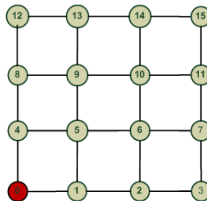
Figure 32 : Topologie maillée
