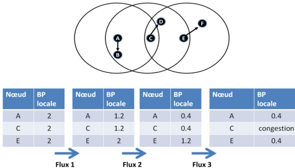
Figure 13 : Blocage du nœud E
