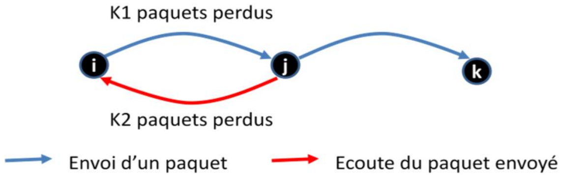
Figure 54: Le nœud i envoie m paquets à j , K_1 sont perdus sur le lien (i, j) . Le nœud j s'il est non mauvais envoie m - K_1 paquets au nœud k et le nœud i entend seulement m - K_1 - K_2 d'entre eux.
