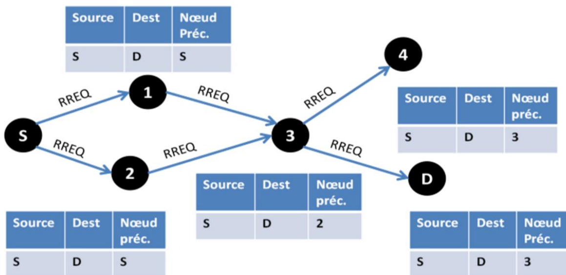
Figure 4 : Broadcaste d'un RREQ par la source S, rediffusé par tous les nœuds qui le reçoivent
