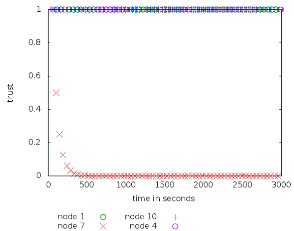
Figure 82 : Confiance des nœuds dans un réseau mesh à topologie en croix avec notre solution lorsque p=0.5
