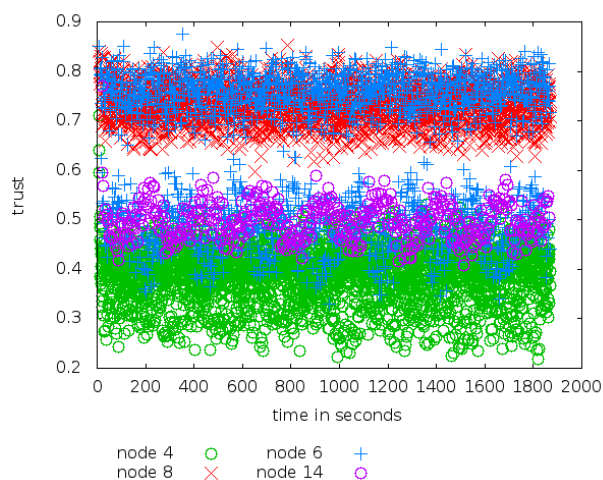
Figure 85 : Confiance des nœuds dans un réseau mesh à topologie maillée avec la solution de référence lorsque p=0.2
