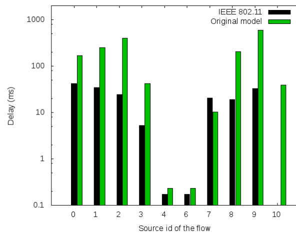
Figure 45 : Délais des flux dans un réseau mesh à topologie chaîné
