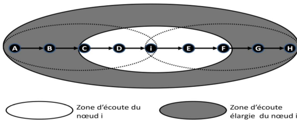
Figure 14 : Zone d'écoute et zone d'écoute élargie d'un nœud
