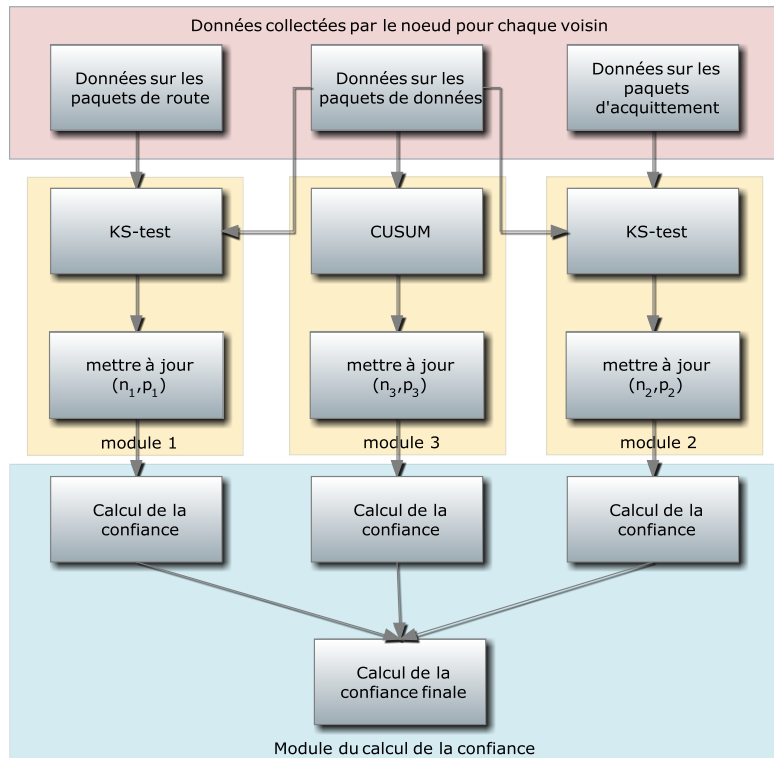
Figure 61 : Système de confiance installé sur chaque nœud du réseau mesh afin d'établir la confiance qu'il a en chacun de ses voisins
