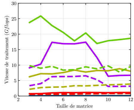
(d) KNL
