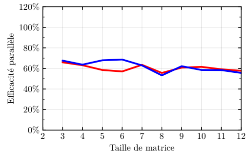
(d) KNL
