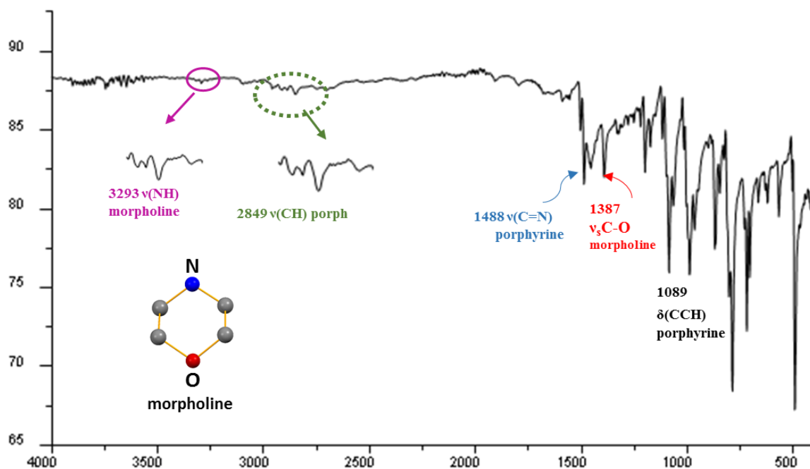
Figure III-15. Spectre IR du [\text{Cd}^{\text{II}}(\text{TCIPP})(\text{morpholine})] (IV) enregistré à l'état solide dans la région [4000-500] \text{ cm}^{-1} .
