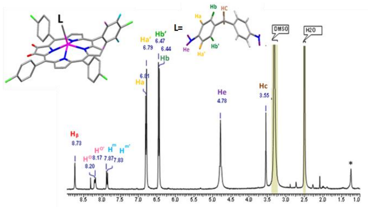
Figure III-9. Spectre RMN ^1\text{H} du complexe [\text{Cd}^{\text{II}}(\text{TCIPP})(4,4'\text{-mda})] ( II ) dans le domaine [1 - 10] ppm. Spectre enregistré à l'ambiante dans le DMSO- \text{d}_6 (* : impuretés), concentration \sim 3 \cdot 10^{-3} M.
