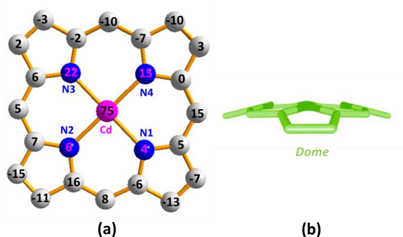
Figure IV-7. (a): Déplacement en ( 10^{-2}\text{Å} ) des atomes par rapport au plan moyen des 24 atomes du Cœur porphyrinique. (b): Schéma d'une distorsion « dome » d'une porphyrine.
