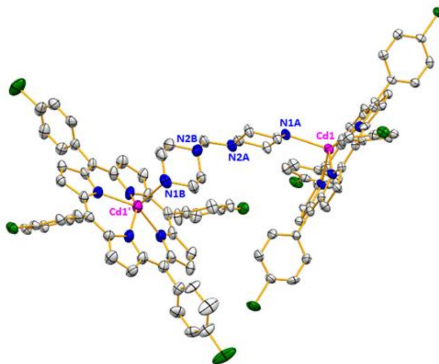
Figure IV-9. Représentation ORTEP de la structure moléculaire du complexe [\{Cd(TCIPP)\}_2(\mu_2\text{-pipyz-CH}_2\text{-pipyz})] (la probabilité des ellipsoïdes est de 40%).
