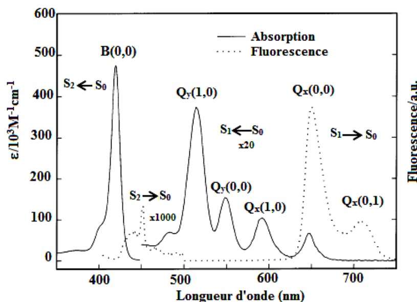
Figure II-16. Spectres d'absorption et d'émission de la porphyrine H_2TPP dans le benzène à 25^\circ C .
