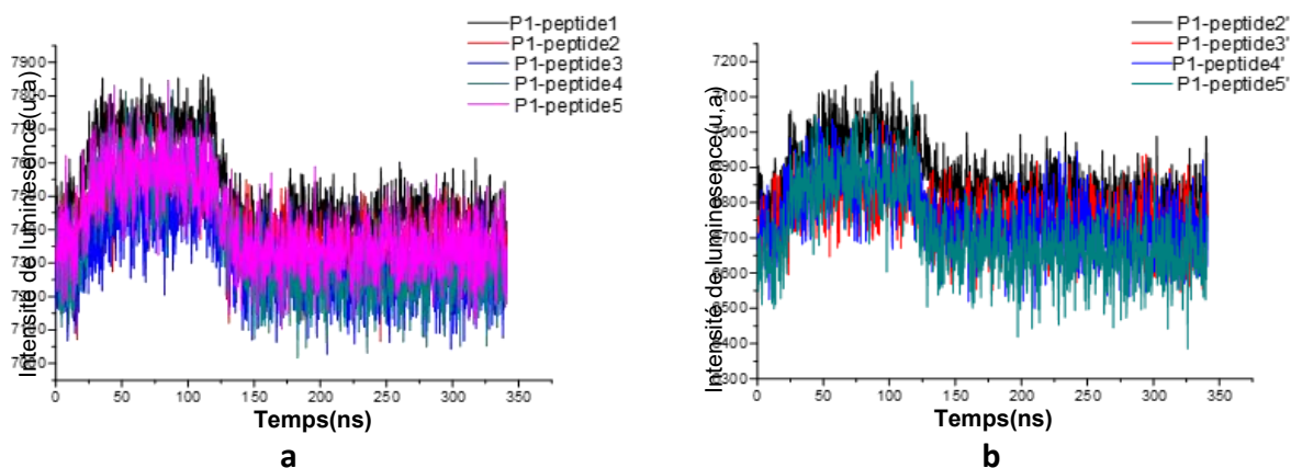
Figure V-18. Spectres de durées de vie d'oxygène singlet. a: Spectres des composés P1-peptide 1-5. b: Spectres des composés P1-peptides 2'-5' .
