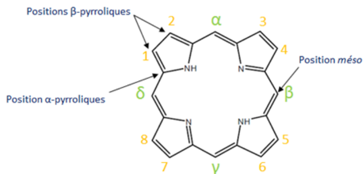
Figure I-3. Système de numérotation de Hans Fischer [28].
