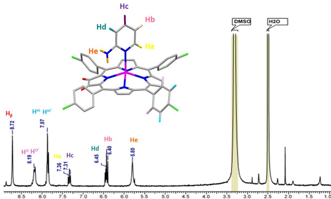
Figure III-8. Spectre RMN ^1\text{H} du complexe [\text{Cd}^{\text{II}}(\text{TCIPP})(2\text{-NH}_2\text{py})](\text{I}) dans le domaine [1 - 10] ppm. Spectre enregistré à l'ambiante dans le \text{DMSO-d}_6 (* : impuretés), concentration \sim 3 \cdot 10^{-3} M.
