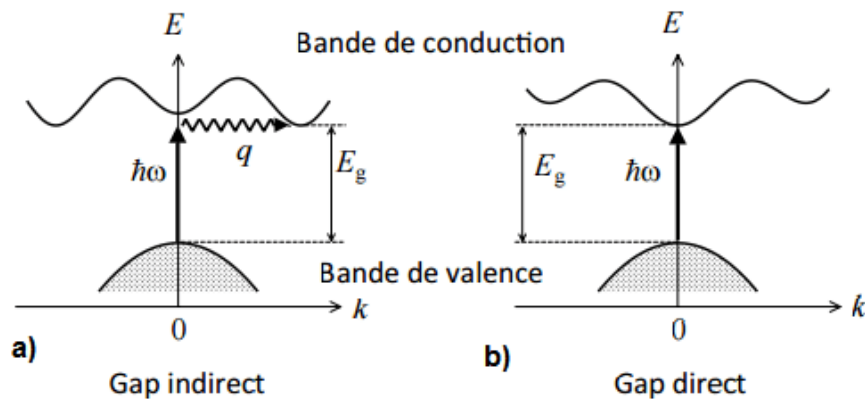
Figure 31 : Diagramme énergétique en fonction du vecteur d'onde k pour un matériau à gap indirect (a) et à gap direct (b) [63].
