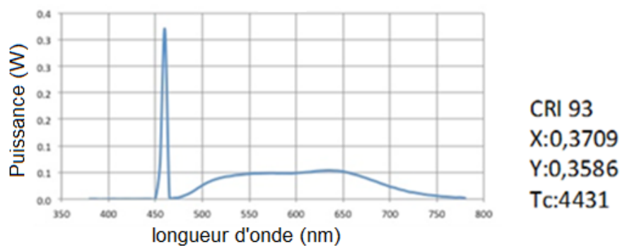
Figure 92 : spectre obtenu pour le couplage de la diode laser avec le luminophore Green YAG 10% en W/(sr/m^2) par nm.
