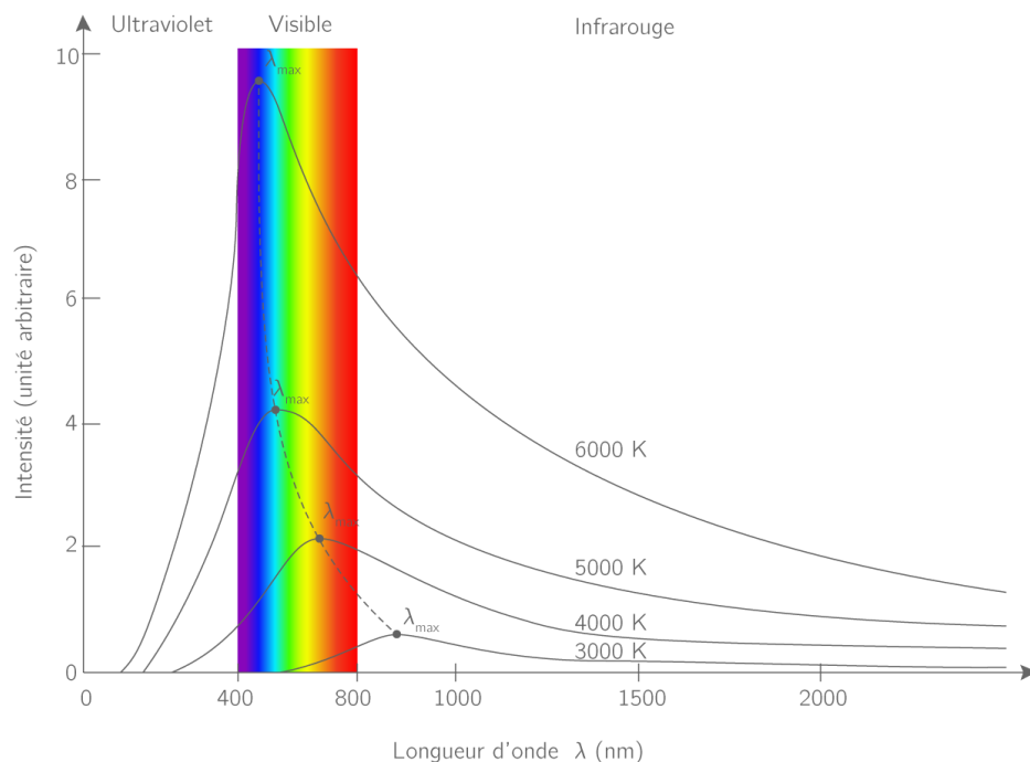
Figure 13 : Description de la théorie des corps noirs.
