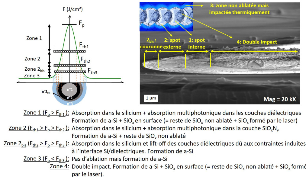
Figure 7: Proposition d'un mécanisme d'ablation laser par "lift-off partiel" en face arrière. Les 5 zones concentriques différemment impactées sont représentées sur les images de microscopie ( F_p = 1.809 \text{ J/cm}^2 , 10% recouvrement, F_{th3} \approx 0.269 \text{ J/cm}^2 ).
