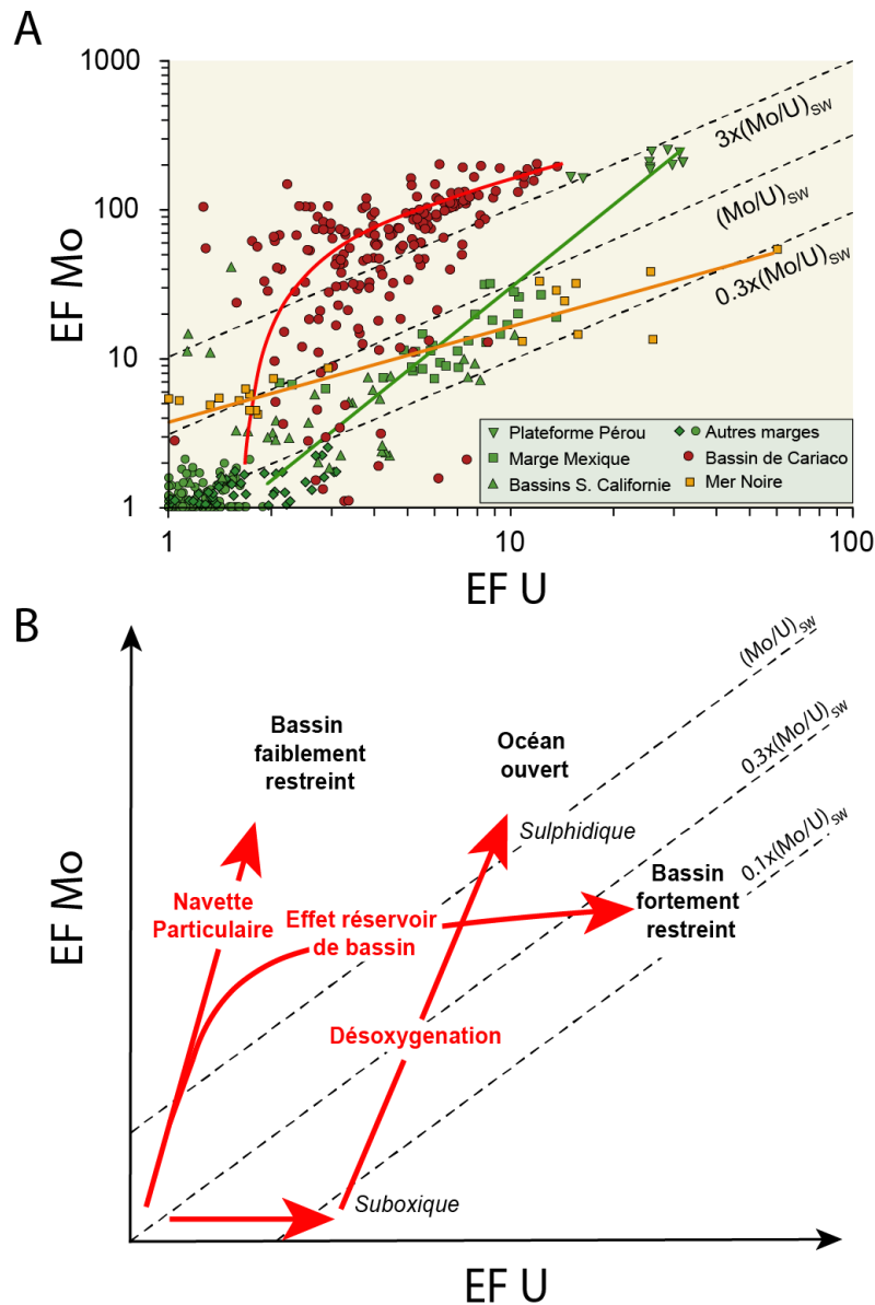
Fig. 6.21 A. Compilations de données provenant de bassins modernes associés à des conditions de désoxygénation (modifié d'après Algeo et Tribovillard, 2009). Les données en vert (Plateforme péruvienne, Bassins du Sud de la Californie, Marge Pacifique du Mexique) représentent des environnements marins ouverts associés à des phénomènes d'upwelling. Les données en rouge correspondent au bassin semi-restreint de Cariaco, celles en orange au bassin fortement restreint de la Mer Noire.
