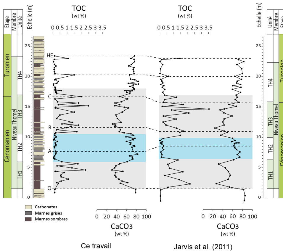
Figure B.6 Corrélation chemostratigraphique basée sur les concentrations en TOC et \text{CaCO}_3 obtenues au cours de ce travail (gauche) et ceux obtenus lors d'études précédentes (droite: Jarvis et al., 2011) à Pont d'Issole. La bande grise correspond à l'intervalle de l'OAE 2 et la bande bleue à l'intervalle du PCE
