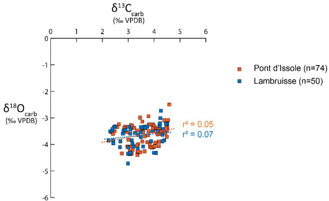
Figure B.1 Rapports \delta^{18}\text{O} et de \delta^{13}\text{C} des carbonates de Pont d'Issole et Lambruisse
