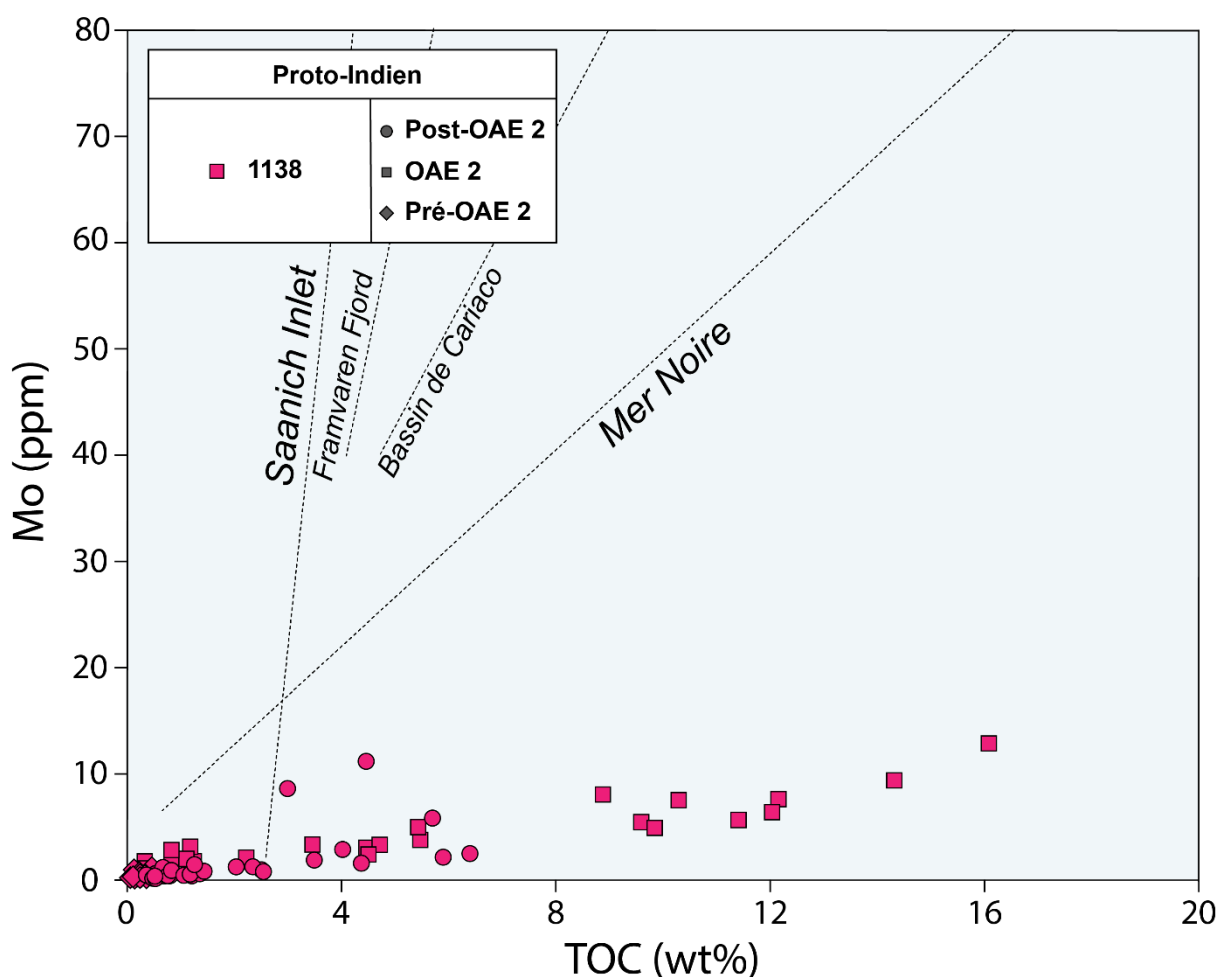
Figure 6.32 Données de concentrations en Mo confrontées aux valeurs de TOC mesurées au niveau du site 1138 (Plateau des Kerguelen)
