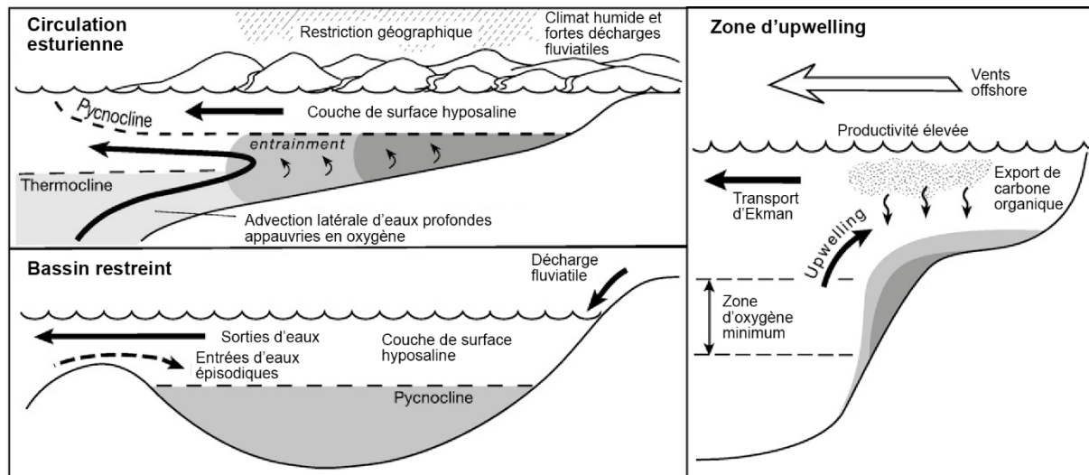
Figure 1.5 Modèles représentatifs des trois modes de mise en place de conditions anoxiques. A. Circulation estuarienne en domaine épicontinental. B. Stratification dans un bassin restreint. C. Zone d'upwelling de marge continentale (d'après Algeo et al., 2008)
