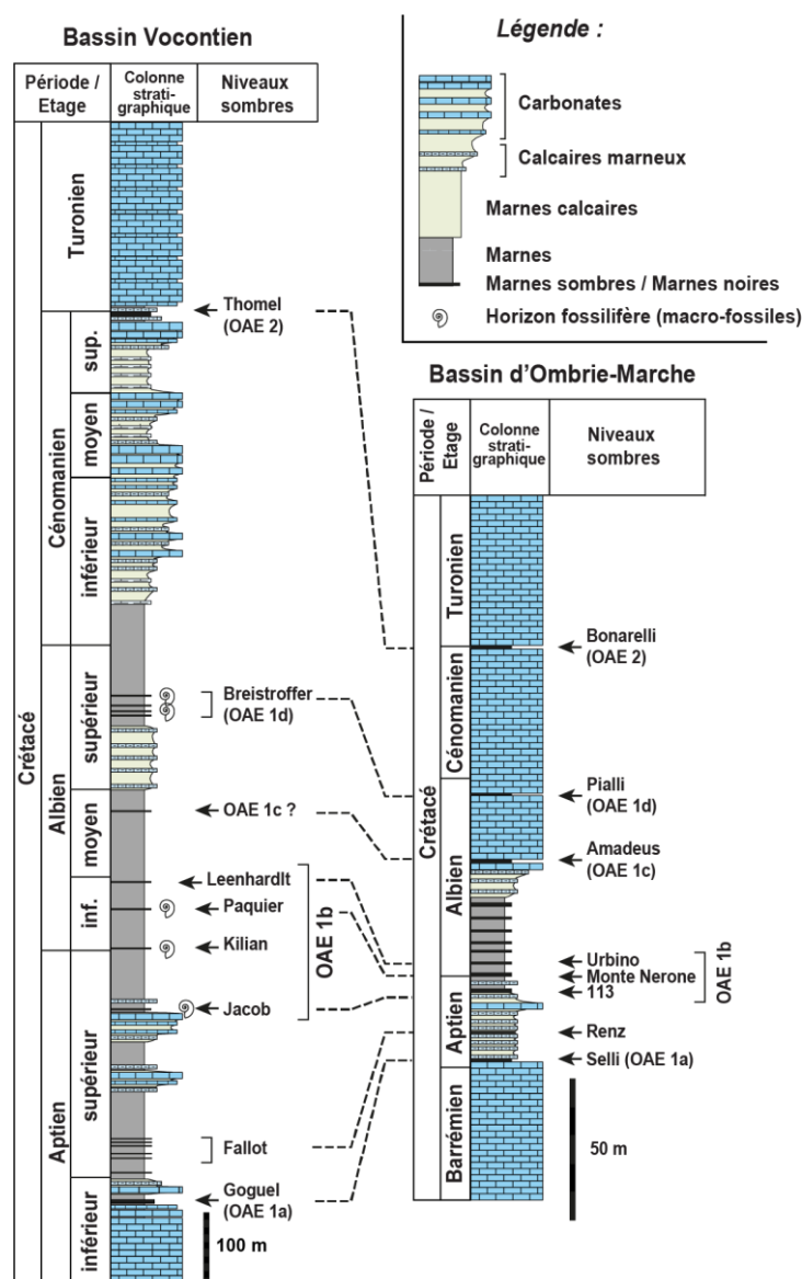
Figure 2.2 Succession stratigraphique du Barrémien au Turonien indiquant la position des niveaux sombres et des événements associés au sein du Bassin Vocontien et du Bassin d'Ombrie-Marche (d'après Takashima et al., 2007)
