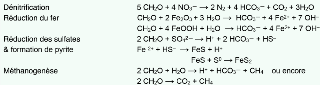
Figure 1.2 Equations des différents processus de dégradation aérobie et anaérobie de la matière organique. Les bilans d'énergies libres de ces réactions ( \Delta G_0 ) sont exprimés en \text{kJ.mol}^{-1} pour des conditions à \text{pH}=7 , température= 25^\circ\text{C} et pression= 1 \text{ bar} )
