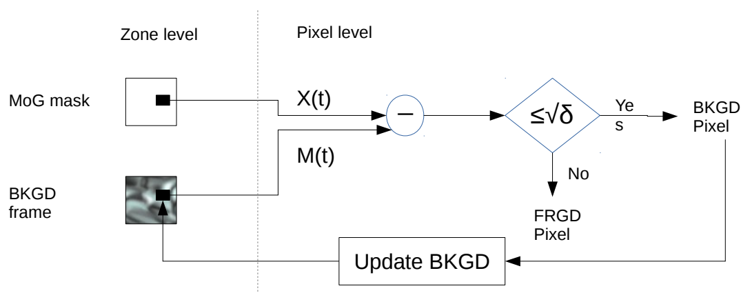
FIGURE 1.6 – Processus de raffinement appliqué sur un pixel dans une zone d'image donnée.
