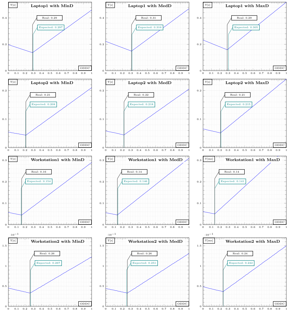
FIGURE 5.12 – Comparaison de l'ODDC estimé avec le temps minimal obtenu sur trois plateformes en utilisant 300 images de chaque dataset présenté sur la Fig. 5.8.
