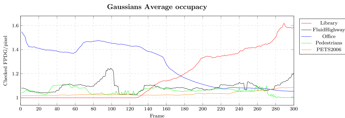
FIGURE 3.4 – Evolution de la dynamique des 300 images les plus significatives de chaque dataset.
