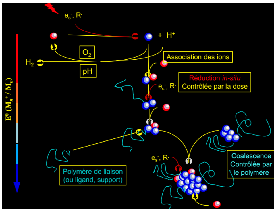
Figure 3 : Agrégats induits par rayonnement. 16 Les atomes (en bleu) formés par réduction des ions (en rouge) par l'électron solvaté ou les radicaux, sont oxydés en présence d'oxygène ou de protons. 16 Pour synthétiser des nanoparticules, il faut donc une atmosphère inerte et un milieu neutre ou légèrement basique. Deux processus de croissance sont possibles, l'un par association des ions avec les atomes et réduction in situ qui n'est pas empêché par les stabilisants (polymère, ligand ou support), l'autre par coalescence entre agrégats qui est fortement inhibée par les stabilisants. Le nombre de germes dépend du débit de dose. À gauche la flèche indique que le potentiel de réduction augmente avec la croissance des agrégats.
