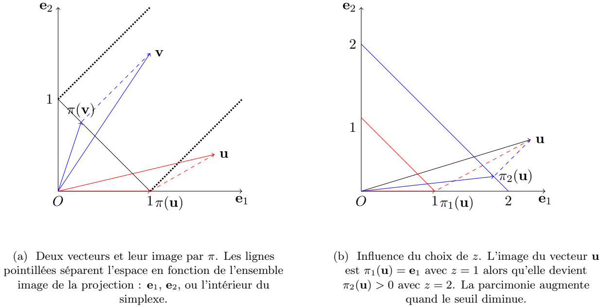
Figure 1: La projection euclidienne sur le simplexe, exemple et influence du choix du seuil.
