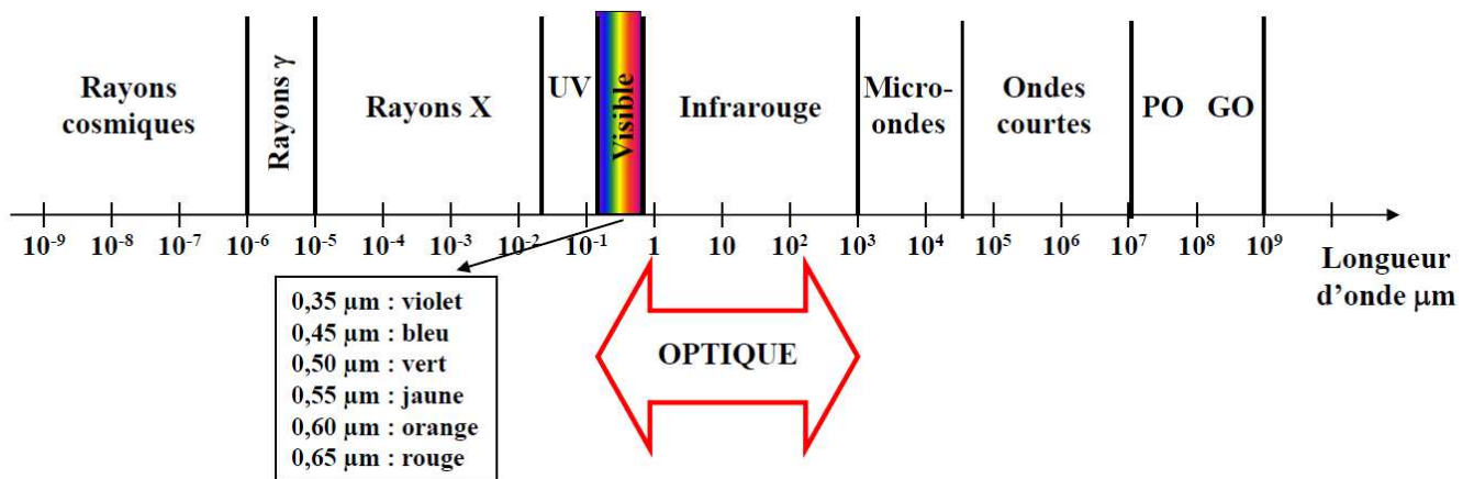
Figure 2.1 : Spectre électromagnétique
