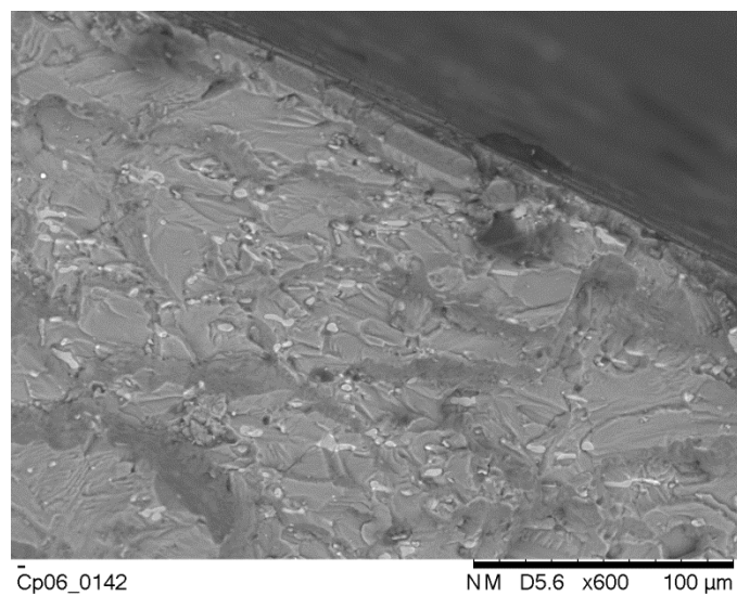
Figure III. 41 : Faciès de rupture d'une éprouvette colmatée, \tau^{\text{alt}} = 170 \text{ MPa} , R_{\tau} = -1 et R_a = 0.8 \mu\text{m}
