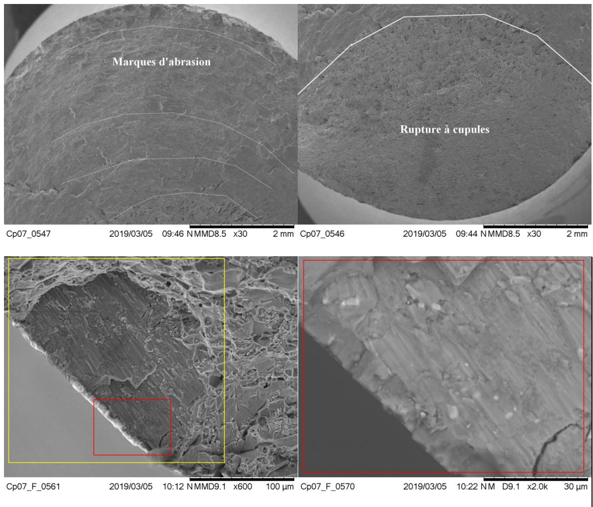
Figure III. 41 : Faciès de rupture d'une éprouvette colmatée, \tau^{\text{alt}} = 170 \text{ MPa} , R_{\tau} = -1 et R_a = 0.8 \mu\text{m}
