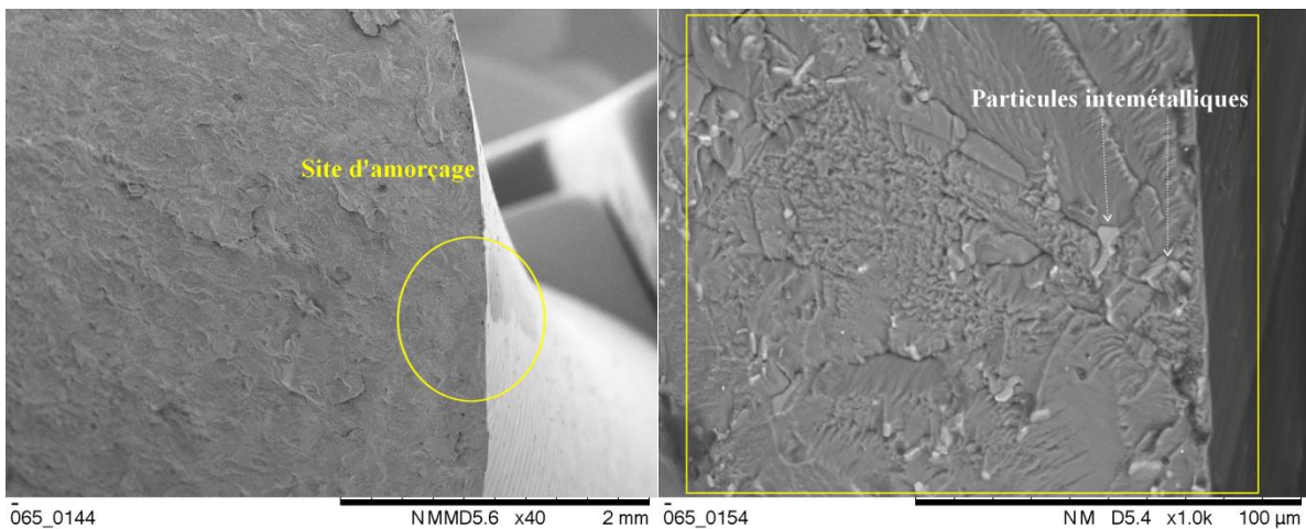
Figure III. 35 : Site d'amorçage d'une éprouvette brute d'usinage testée en torsion ( \tau^{\text{alt}}=70 MPa, R_{\tau}=0.1 et R_a=0.8 \mu\text{m} )
