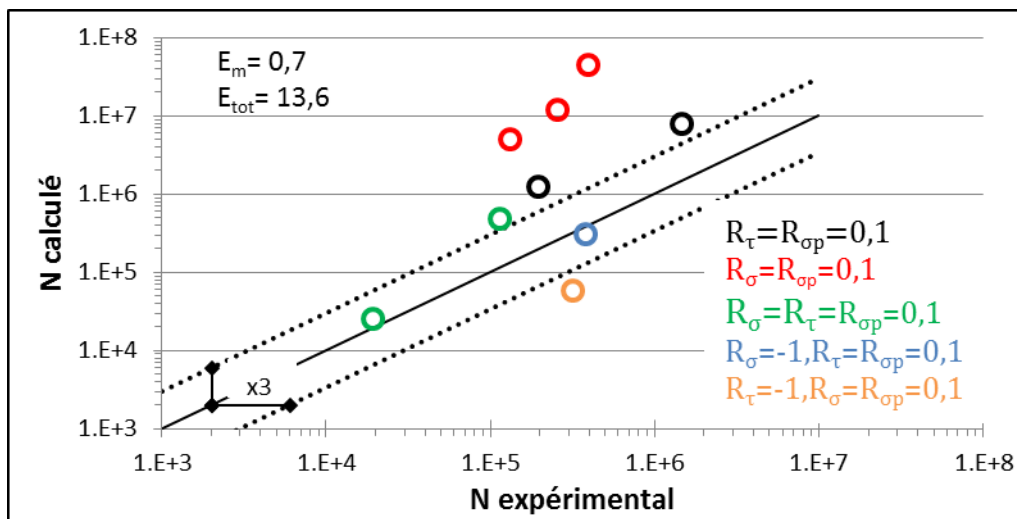
Figure V. 17 : Nombre de cycles à rupture Vs nombre de cycles expérimental en traction et/ou torsion et pression interne combinée-Modèle de Fatemi-Socie
