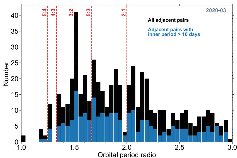
FIGURE 2.4 – Histogramme du rapport de période orbitale entre chaque paire adjacente de planètes parmi les systèmes multi-planétaires confirmés par Kepler (noir). L'histogramme bleu concerne uniquement les paires adjacentes de planètes pour lesquelles la planète interne a une période orbitale excédant 10 jours. Figure adaptée de Baruteau & Papaloizou (2013) avec les données extraites de exoplanet.eu .
