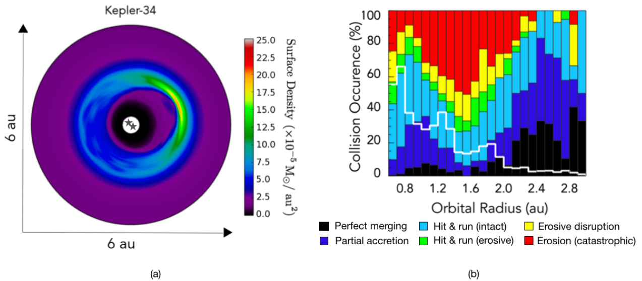
FIGURE 2.7 – (a) Densité surfacique de gaz dans une simulation hydrodynamique 2D modélisant le disque circumbinaire autour de l'étoile Kepler-34, où l'on constate que les parties internes du disque acquièrent une excentricité assez large à cause de la proximité de la binaire. Figure tirée de Lines et al. (2015) . (b) Impact des collisions entre planétésimaux dans une simulation à N corps incluant une modélisation simplifiée du gaz du disque circumbinaire autour de Kepler-34. Figure tirée de Lines et al. (2016) .
