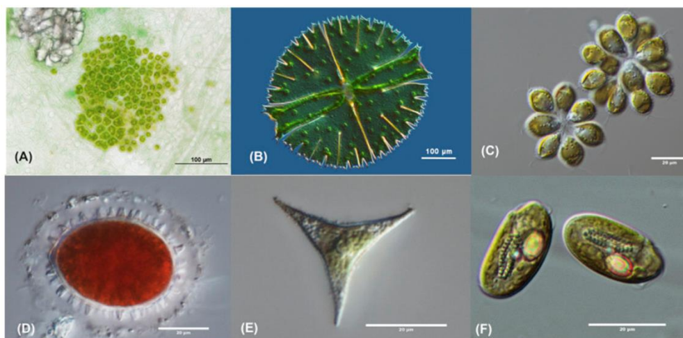
Figure 23 : Illustration d'une partie de la diversité des microalgues. (A): Colonie de Pediatrum sp. ; (B): Micrasterias radiosa ; (C): Synura petersenii ; (D): Chlamydomonas sp. ; (E) Pseudogoniochloris tripus ; (F) Cryptomonas sp. (Adapté de Borowitzka, 2018).
