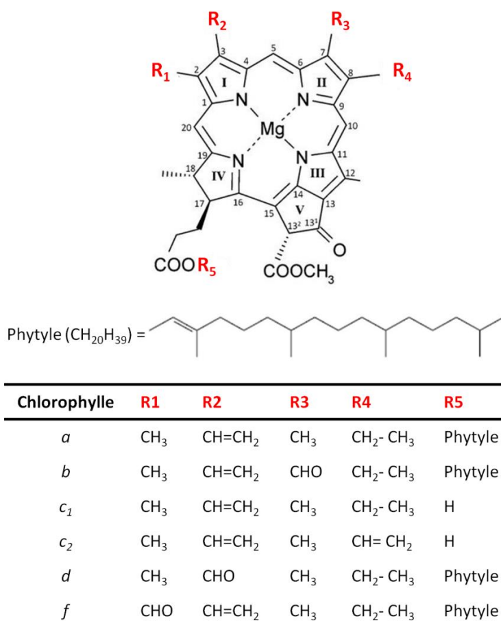
Figure 27 : Formules structurales des chlorophylles. (Adapté de Voloshin et al., 2015; Moraçais et al., 2018).
