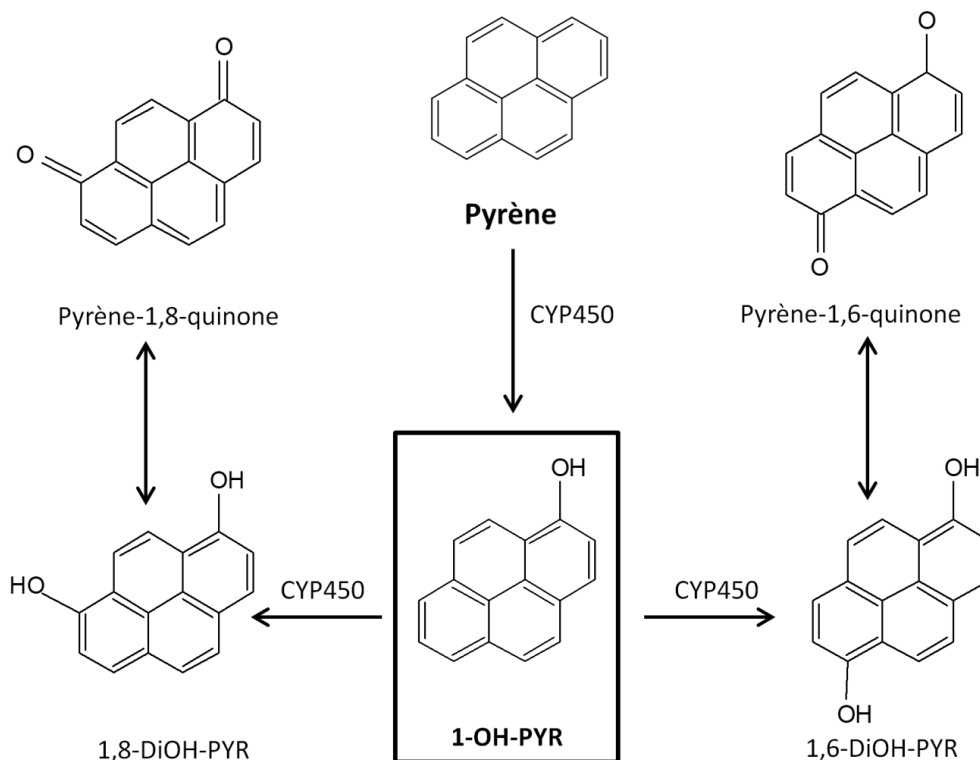
Figure 14 : Métabolisme du pyrène en 1-hydroxypyrrène (1-OH-PYR) et son oxydation ultérieure en pyrène-1,6- et 1,8-quinone par l'intermédiaire du 1,6- et 1,8-dihydroxypyrrènes (DiOH-PYR). (Adapté de Lotz et al., 2016).
