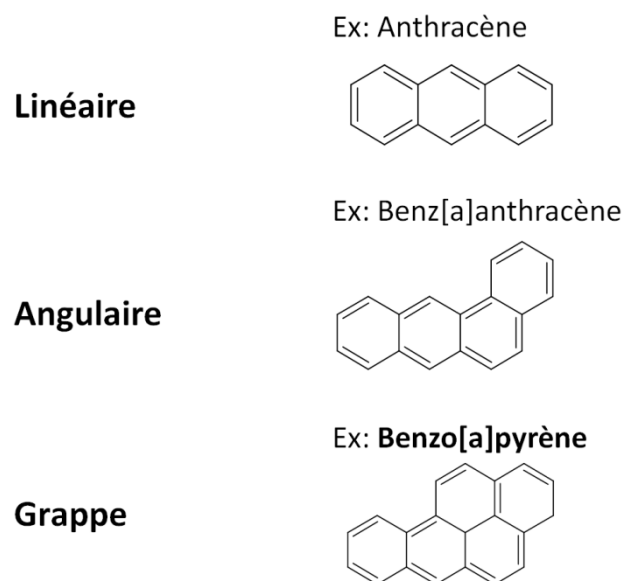
Figure 1 : Disposition moléculaire des hydrocarbures aromatiques polycycliques. (Adapté de Edwards, 1983; Abdel-Shafy and Mansour, 2016).
