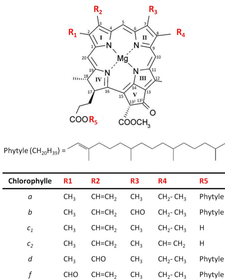
Figure 27 : Formules structurales des chlorophylles. (Adapté de Voloshin et al., 2015; Morançais et al., 2018).
