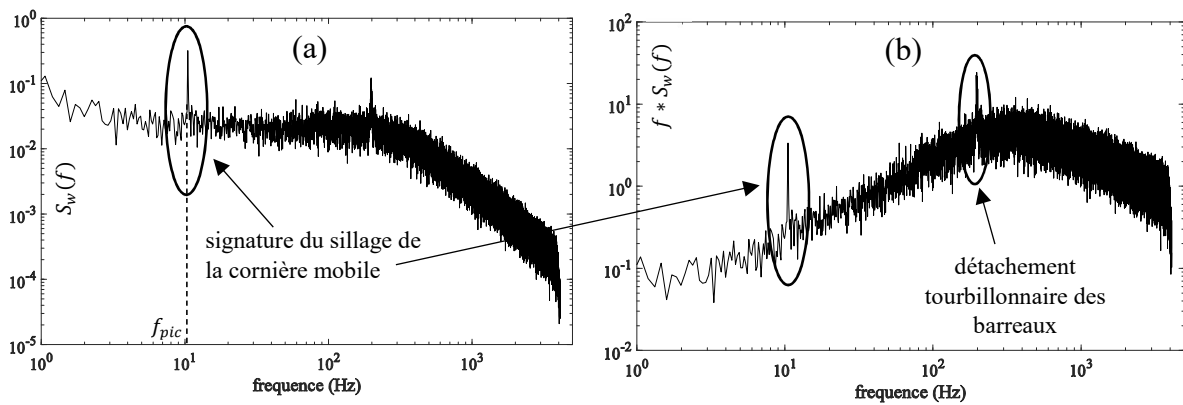
Figure 127. (a) Densités spectrales de puissance du vent turbulent généré par le montage avec \bar{U} = 13,1 \text{ m/s} , f_e = 10,5 \text{ Hz} . (b) La même DSP multipliée par la fréquence
