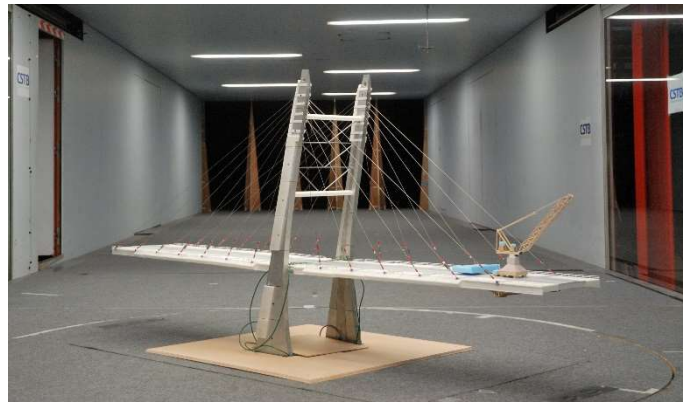
Figure 57. La maquette aérodynamique du pont de Korabelny à Saint-Petersbourg en construction, © CSTB
