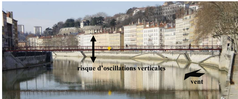
Figure 32. La passerelle suspendue sur la Saône à Lyon
