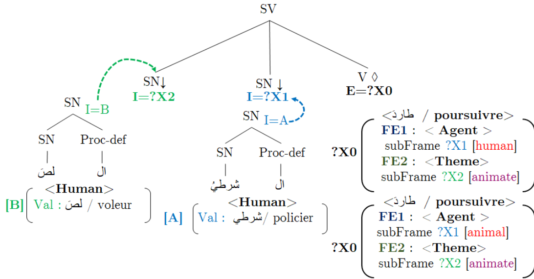
FIGURE 4.35: Processus de l'analyse syntaxico-sémantique de la phrase
