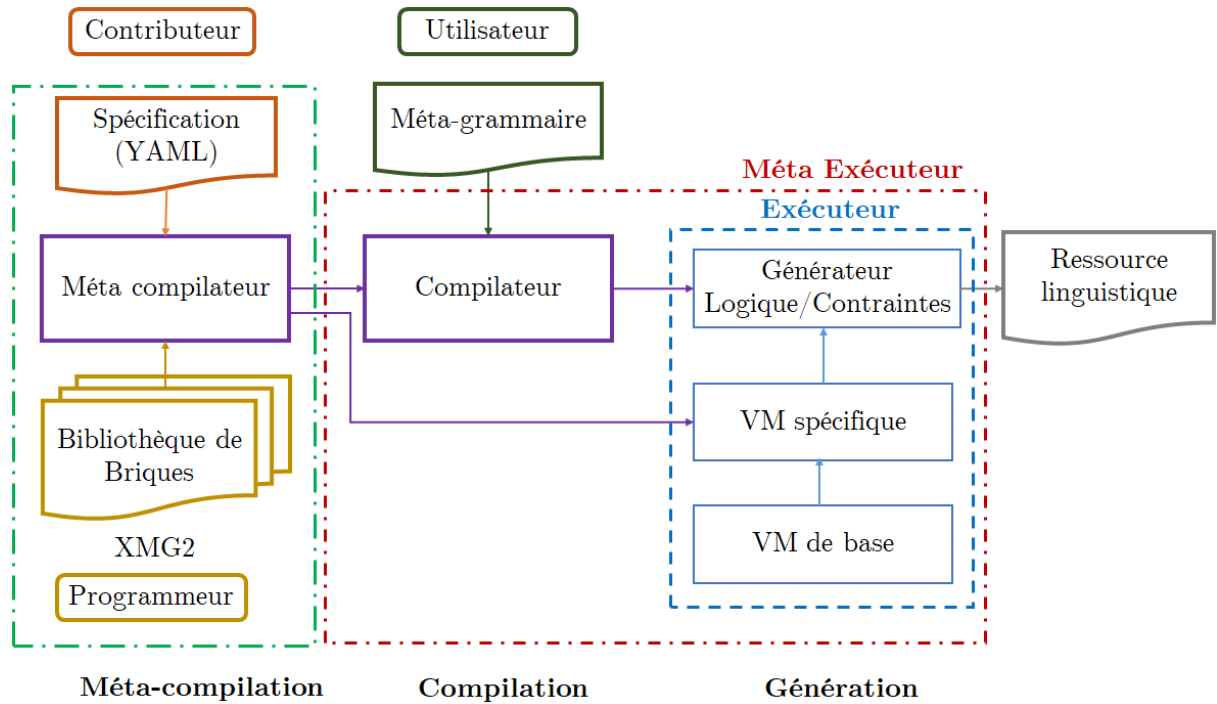
FIGURE 3.7: L'architecture modulaire de XMG2
