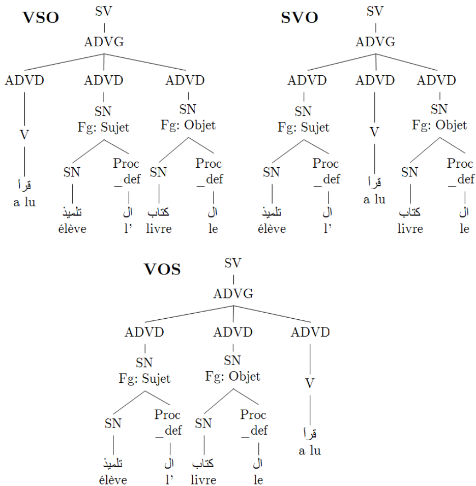
FIGURE 4.8: Ordre de mot libre de la phrase (L'élève a lu le livre)
