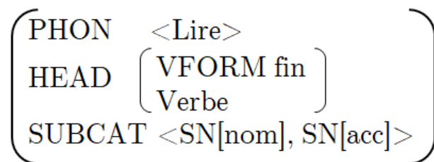
FIGURE 1.13: Exemple de l'entrée lexicale "Lire"
