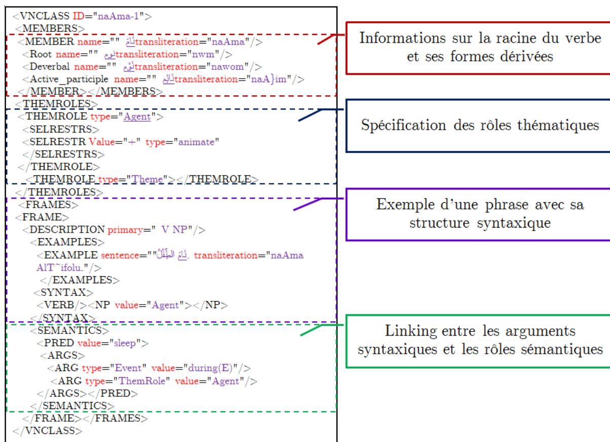
FIGURE 2.12: Extrait du fichier XML de la classe naAma (dormir) dans ArabicVerbNet
