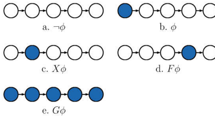
FIGURE 2.14 – Représentation de la logique temporelle linéaire
