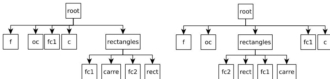
a. Graphe de scène enrichi du code 4.2 b. Graphe de scène enrichi du code 4.3
