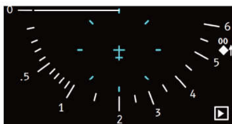
FIGURE 6.7 – Affichage du TCAS intégré à l'IVSI ne vérifiant pas l'exigence E_5
