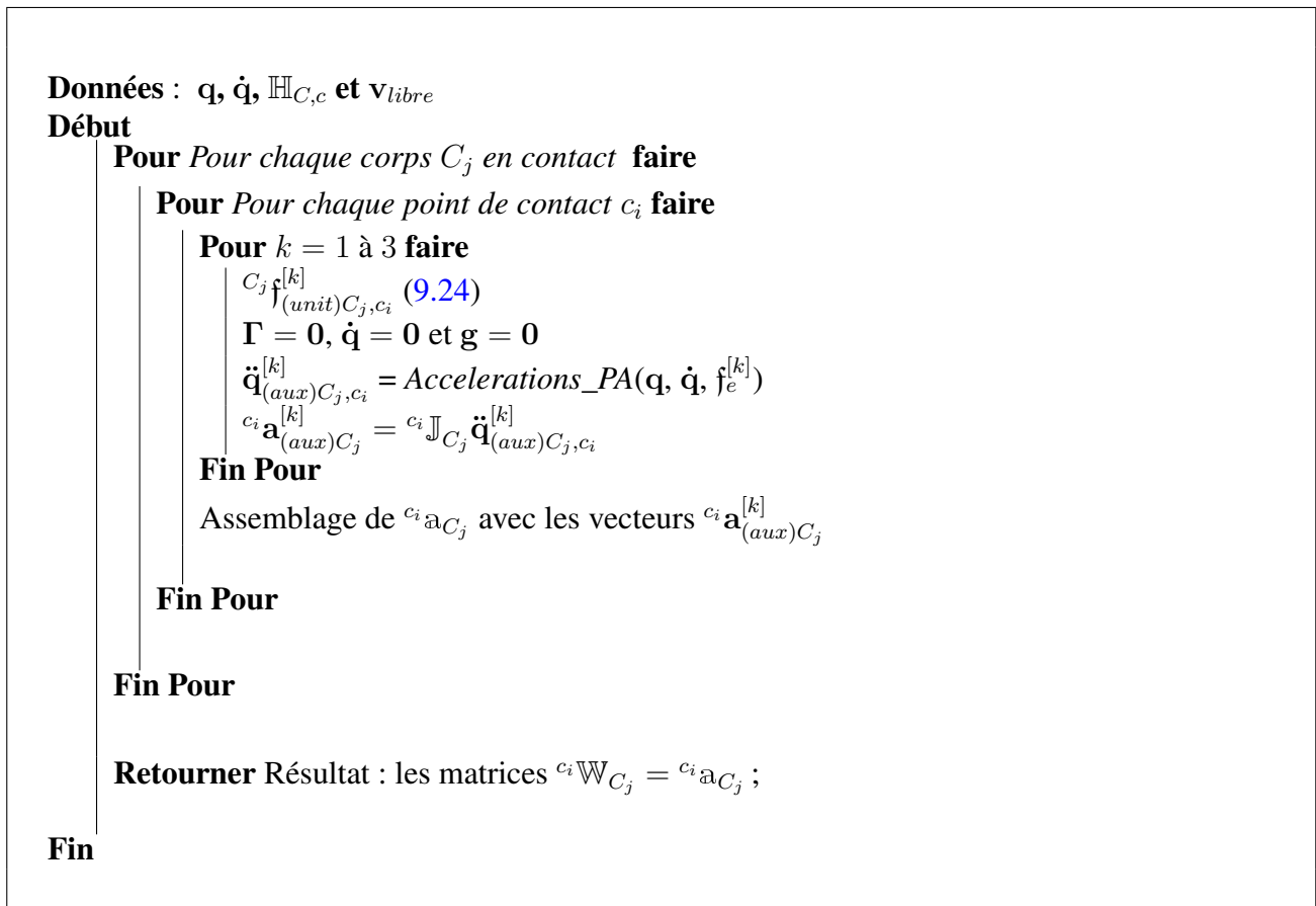
Algorithme 4 – Algorithme de calcul de la matrice de Delassus {}^c \mathbb{W}_C
