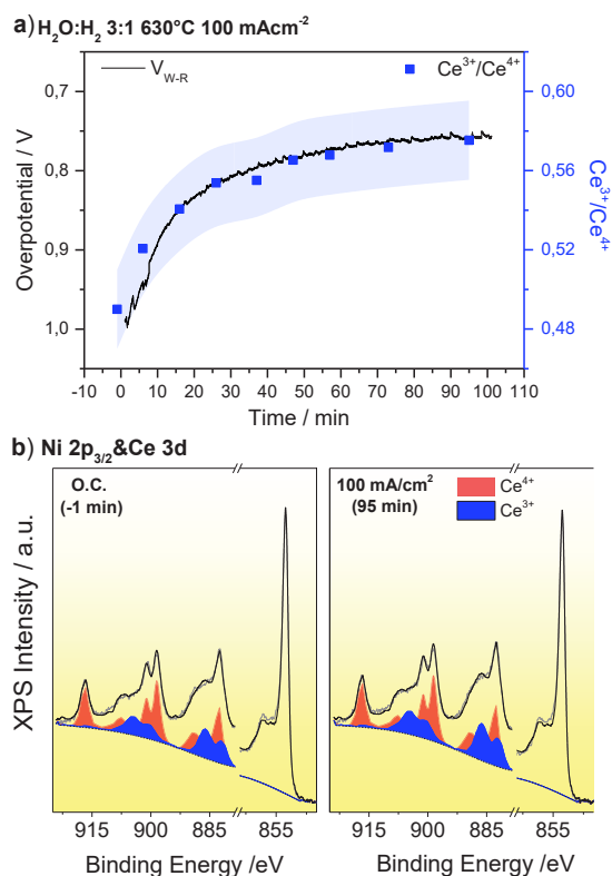
Figure 1. Réduction de l'électrode Ni-GDC a) Évolution dans le temps du surpotentiel de cellules Ni-GDC / YSZ / Pt (ligne noire continue) et évolution du rapport des composants \text{Ce}^{3+} / \text{Ce}^{4+} (points bleus), déduite de l'analyse des spectres 3d correspondants de NAP-XPS Ce. Les mesures ont été effectuées sur des cathodes Ni-GDC pré-oxydées dans un mélange gazeux \text{H}_2\text{O} / \text{H}_2 3: 1 à 640 ° C et à courant constant de -100 mA / cm 2 . Le fond bleu représente l'incertitude dans le calcul du ratio \text{Ce}^{3+} / \text{Ce}^{4+} principalement lié à la procédure de désomation. b) Spectres NAP-XPS caractéristiques de Ni2p 3/2 et Ce 3d dans \text{H}_2\text{O} / \text{H}_2 avant et après l'application en cours. Deux composantes de Ce 3d ont été utilisées pour ajuster les spectres correspondant aux états d'oxydation \text{Ce}^{3+} (bleu) et \text{Ce}^{4+} (rouge) de l'oxyde de cérium.
