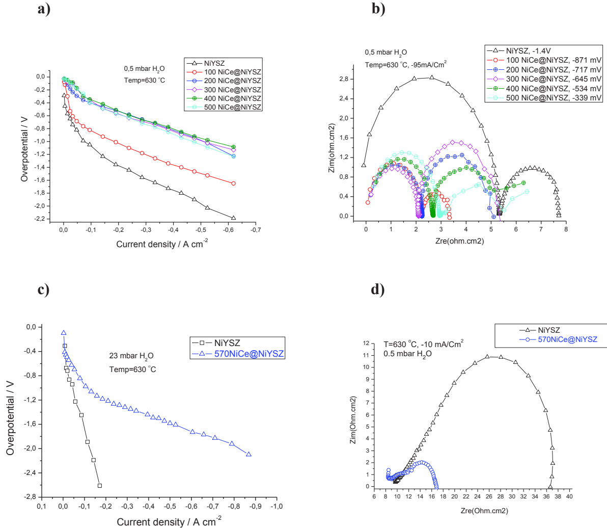
Figure 5. a) Courbes de densité de surtension du courant mesurées dans des conditions d'électrolyse à la vapeur (à 650 °C sous 0.5 mbar de 100% \text{H}_2\text{O} ) sur des électrodes Ni-YSZ avant et après l'addition de deux imprégnations de NPs \text{Ni}_{0,1}\text{Ce}_{0,9}\text{O}_{2-x} (100, 200, 300, 400, et 500 et 570 \mu\text{L} ). b) Les données d'impédance sont indiquées ci-dessus pour chaque charge d'électrodes de travail Ni-YSZ et NiCe@NiYSZ. c) Courbes de densité de surtension du courant mesurées sur des électrodes de travail NiYSZ et 570NiCe@NiYSZ (pour une imprégnation de 570 \mu\text{L} lors d'une électrolyse de tige à 650 °C à 23 mbar 100% \text{H}_2\text{O} ). d) Données d'impédance correspondantes des électrodes de travail. Une électrode Un compteur de Pt et des électrodes de référence de géométrie identique ont été utilisés dans toutes les mesures.
