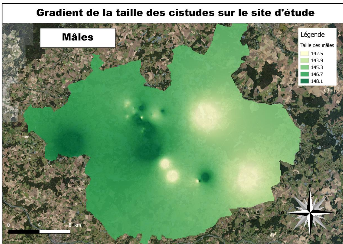
Figure 48 : Répartition de la taille des mâles sur le site d'étude
