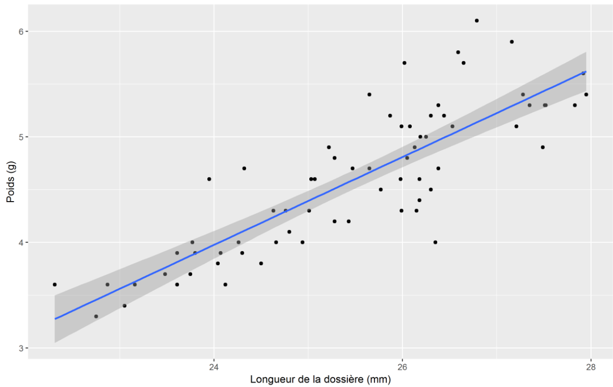
Figure 29 : Relation entre le poids et la longueur de la dossière des émergents
