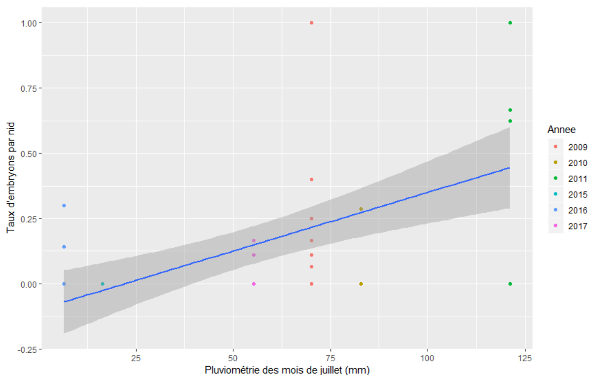
Figure 28 : Taux d'embryons avortés en fonction de la pluviométrie du mois de juillet
