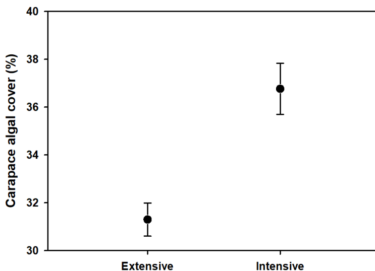
Figure 60 : Couverture algale selon le type de pisciculture
