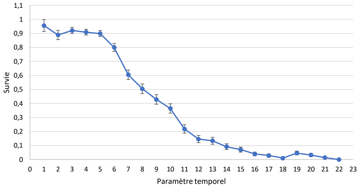
Figure 43 : Taux de survie au cours du temps ( \pm ET ) (Paramètre temporel : une unité correspond à 5 jours, Barbraud, com. pers.)
