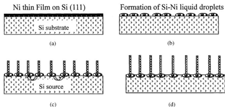
Fig. 7 : Schéma de principe de la croissance SLS 3D de nanofils de silicium par proced SLS utilisant le nickel comme catalyseur
