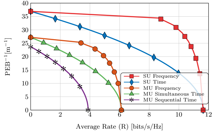
FIGURE 5: Illustration du compromis entre l'inverse de la borne théorique d'erreur de positionnement, PEB, et le débit de données moyen, R , pour diverses stratégies de répartition des ressources en fréquence et en temps et pour des scénarios mono- et multi-utilisateurs (chaque courbe est iso-budget).
