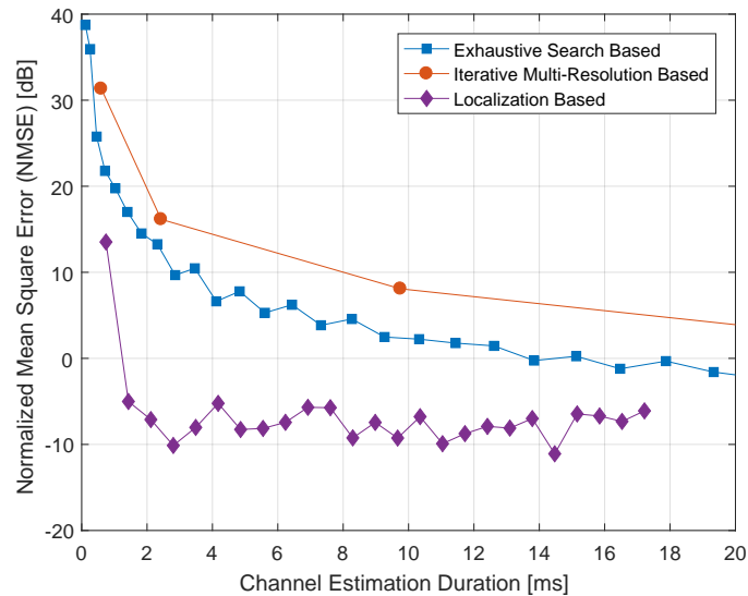
FIGURE 10: Erreur quadratique moyenne normalisée (NMSE) d'estimation du canal multi-trajets mmWave pour la méthode proposée s'appuyant sur l'information de localisation et deux méthodes de recherche conventionnelles, en fonction de la durée.
