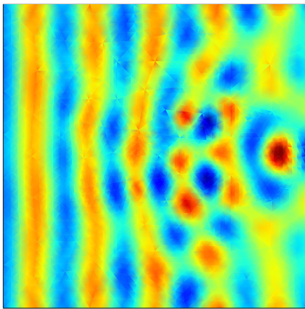
(d) DGT solution on M2 (21690 d.o.f.)
