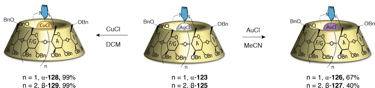
Scheme II-12: Synthesis of (α-ICyD)CuCl, (α-ICyD)AuCl, (β-ICyD)CuCl and (β-ICyD)AuCl
