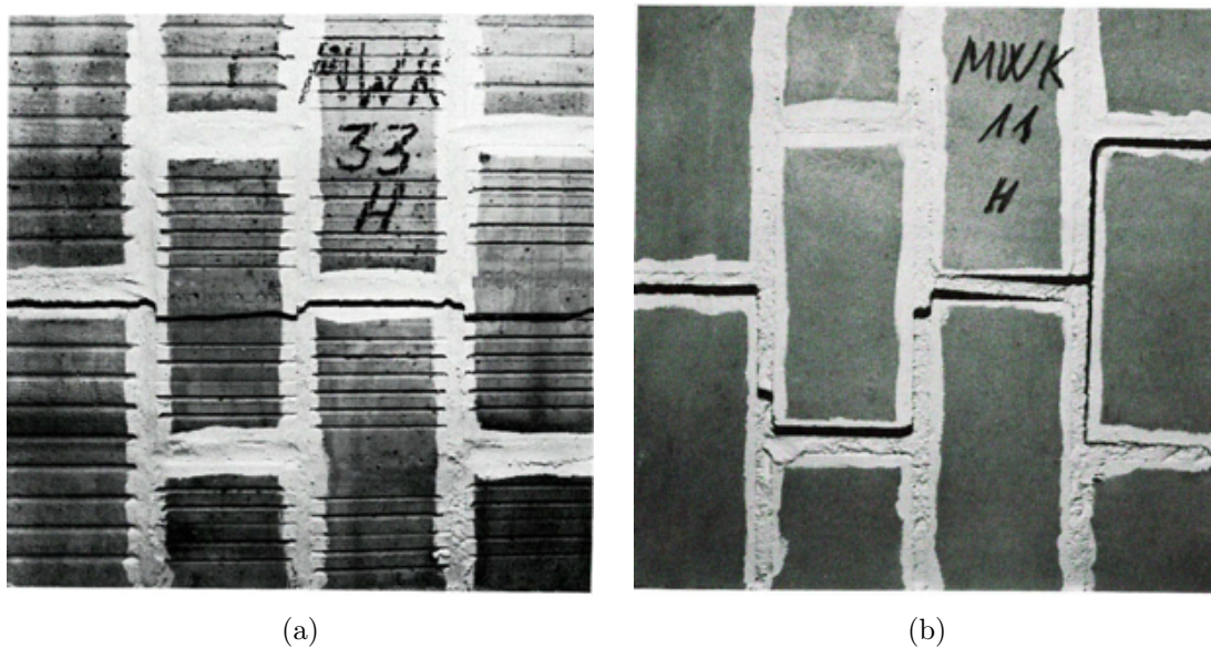
FIGURE 1.21 – Mécanismes de ruine observés pour une sollicitation parallèle aux lits de mortier [Fig. 1.20a] : (a) Cas 1 et (b) Cas 2 (Backes, 1985)
