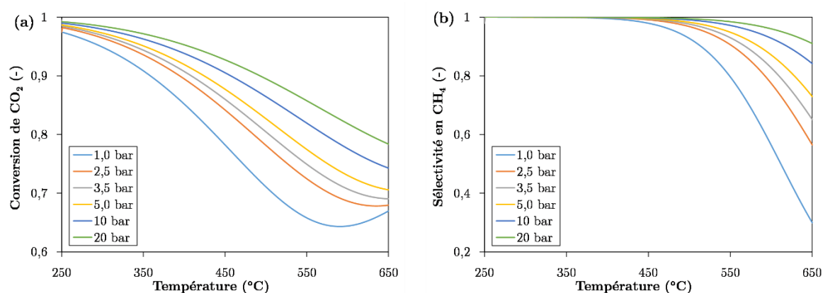
Figure I.2 – (a) Evolution du taux de conversion de CO 2 et (b) évolution de la sélectivité en CH 4 à l'équilibre thermodynamique en conditions stœchiométriques en fonction de la température et de la pression
