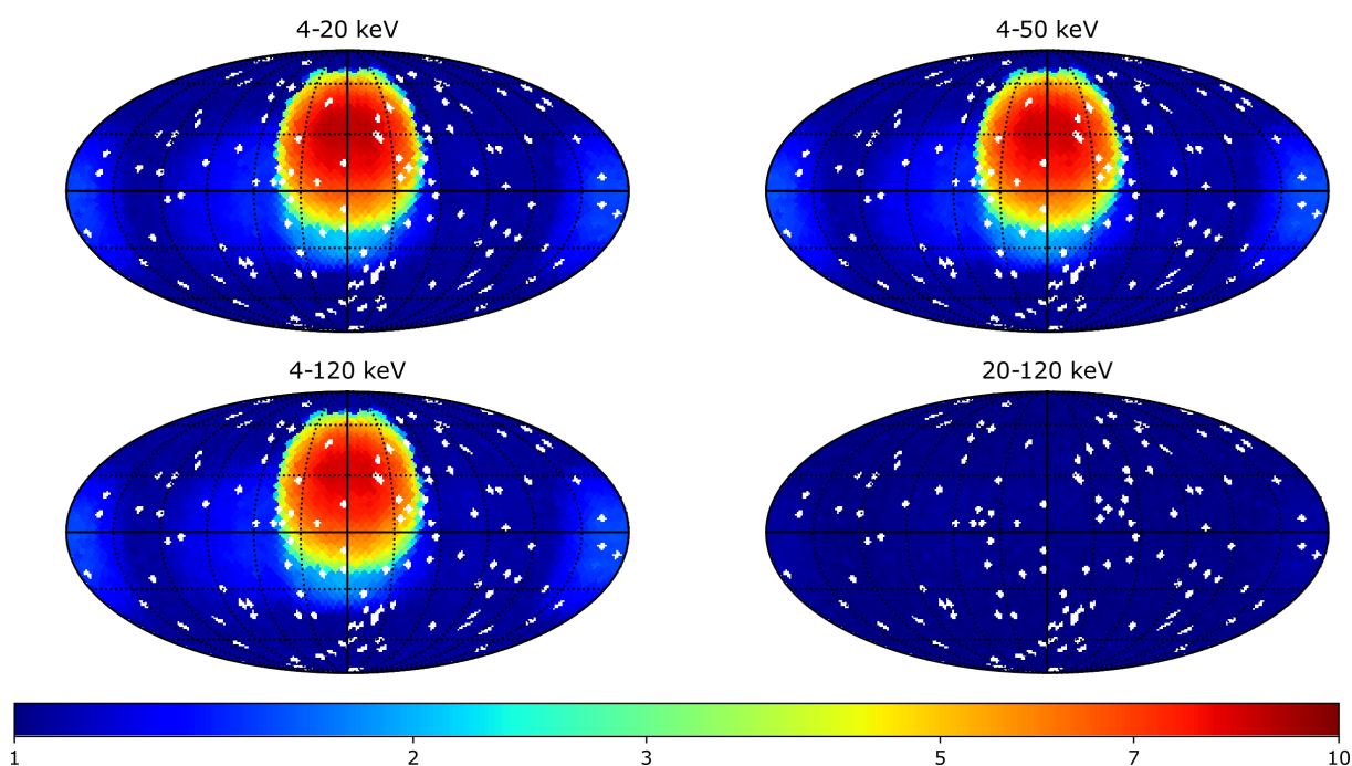
Figure 4.19 – Influence des sources du catalogue sur les images du ciel : écart-type de la distribution du SNR dans les images du ciel de 20 s selon la direction de pointage dans le ciel en coordonnées galactiques (longitude croissante de droite à gauche). Les quatre cartes correspondent aux bandes d'énergie prévues pour l'algorithme de déclenchement embarqué.
