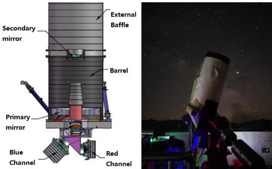
Figure 2.7 – Gauche : design du télescope VT. Droite : modèle de qualification en test à l’observatoire de Xinglong (Chine).
