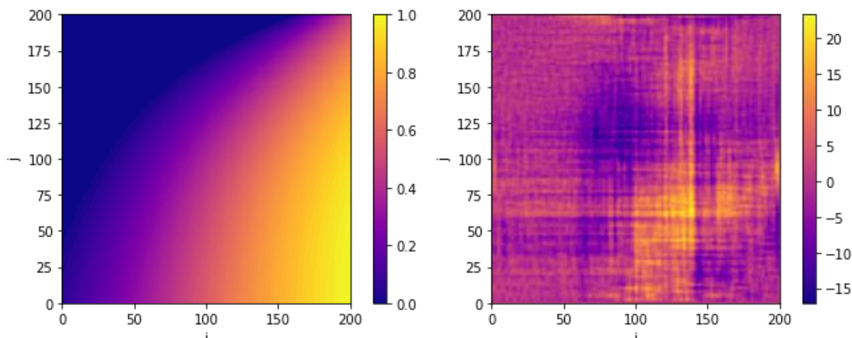
Figure 4.5 – A gauche : carte d'exposition du ciel normalisée pour une exposition de 20 min (position et attitude du satellite mis à jour toutes les minutes pendant les 20 premières minutes de l'année de la simulation du CNES). Dans cette simulation, la Terre quitte peu à peu le champ de vue. La couleur donne la fraction d'occultation de chaque pixel par la Terre. A droite : image du ciel en SNR pour la plus longue durée d'exposition prévue à bord (1310.72 s). Simulations réalisées avec redistribution en énergie et détection dans la bande 4–120 keV (énergies injectées dans 4–150 keV) sans correction du bruit de fond.
