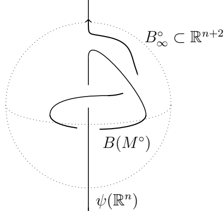
FIGURE 3.1 – Un nœud long dans l'espace M^\circ . La boule (en pointillé) représente B(M) . Son extérieur est B_\infty^\circ , contenu dans \mathbb{R}^{n+2} .
