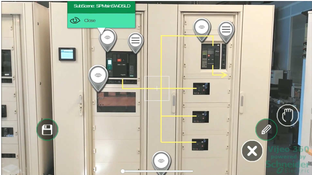
FIGURE 2.5 – Interface de l’application de RA Vijeo : schéma électrique superposé à la machine et reliant plusieurs POIs
