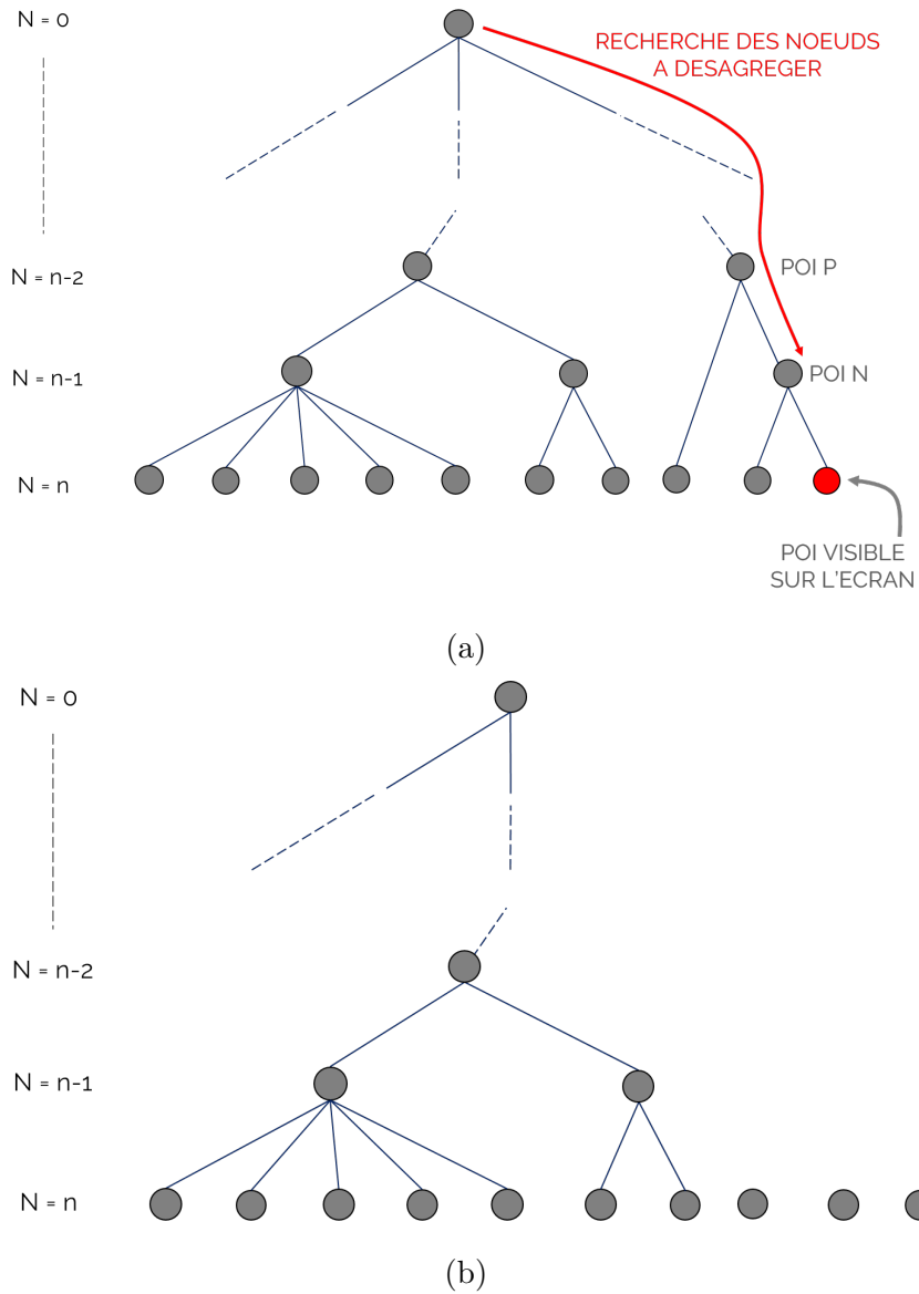
FIGURE 4.12 – Processus de désagrégation. a) Recherche des nœuds dont les halos fils ne se chevauchent plus ou n’existent plus. b) Élimination des parents du nœuds désagrégés.
