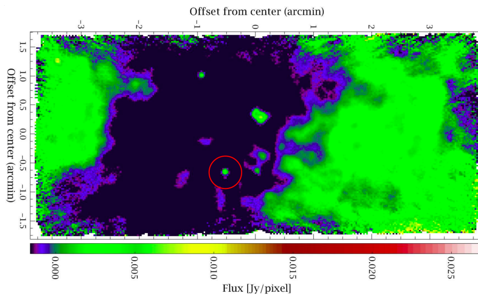
FIGURE 9.6 – Champ de vue Herschel /PACS dans la région d’IGR J16318-4848 à 70 \mu\text{m} . IGR J16318-4848 est entourée en rouge. Source: Herschel Science Archive, ESA
