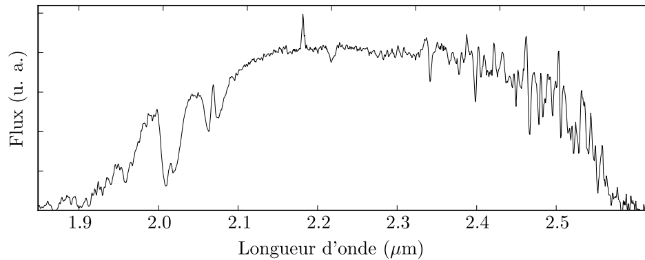
(b) Spectre corrigé par Molecfit.
