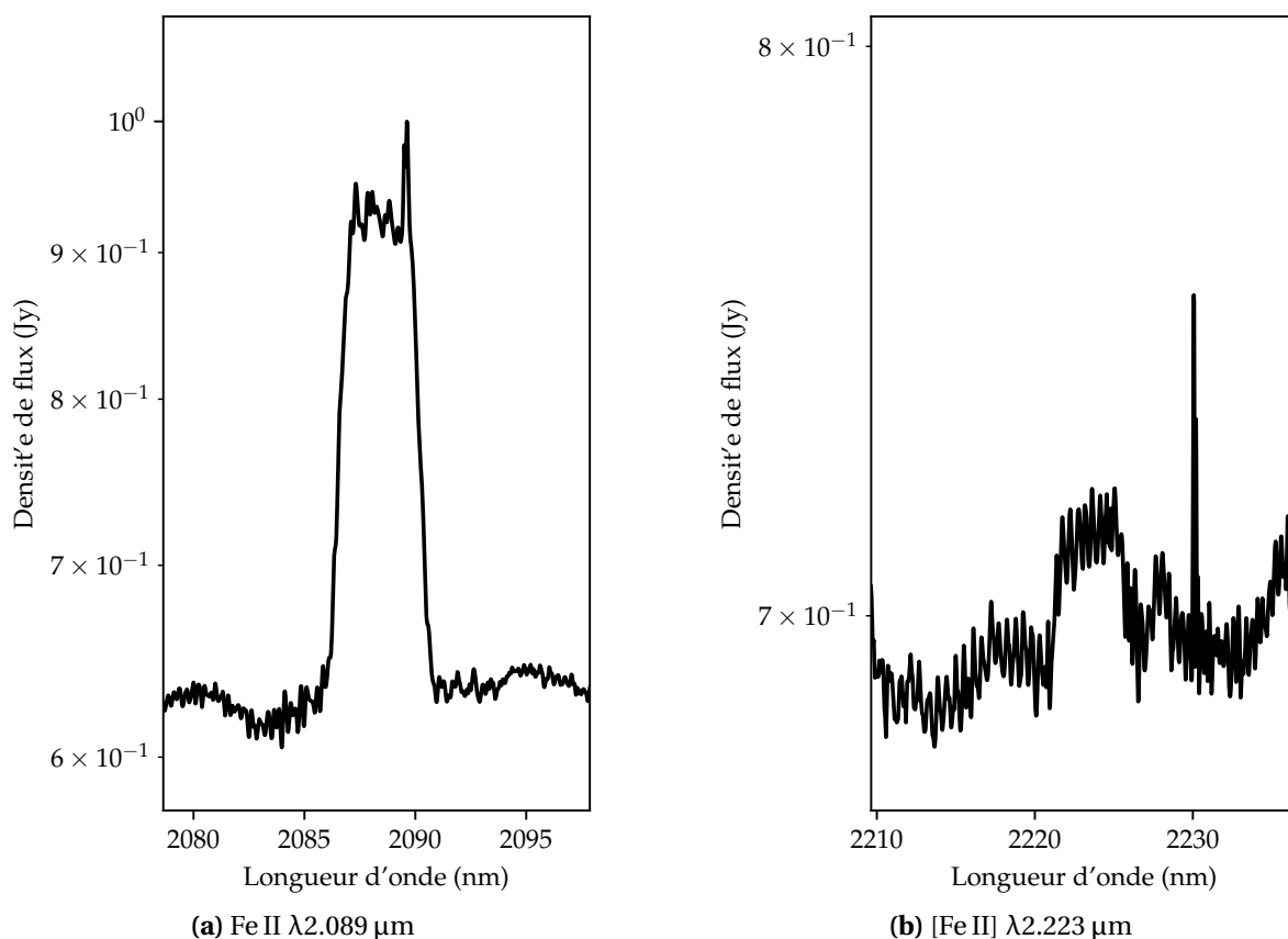
FIGURE 10.3 – Exemple de deux raies du fer en plateau. Données issues du spectre NIR d'X-Shooter.
