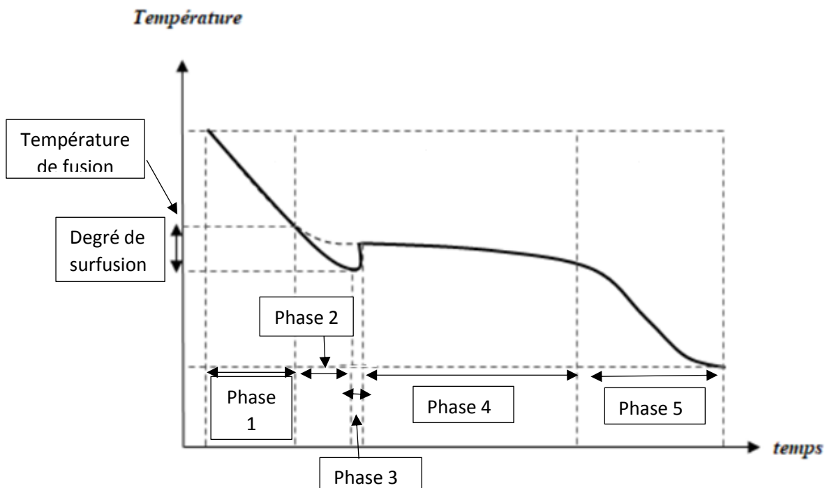
Figure 65 : Evolution de la température en fonction du temps, pour un matériau présentant une surfusion [98].
