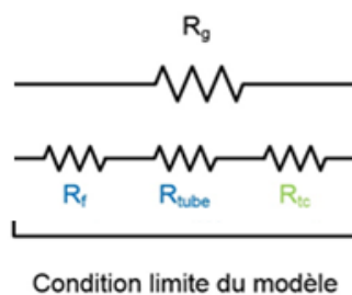
Figure 187 : Schéma des résistances thermiques en série
