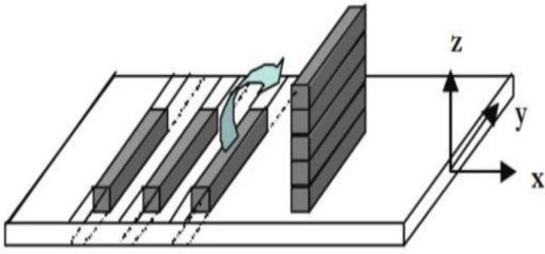
Figure 77 : Découpe des échantillons pour la mesure de la conductivité thermique dans la direction plane [101].
