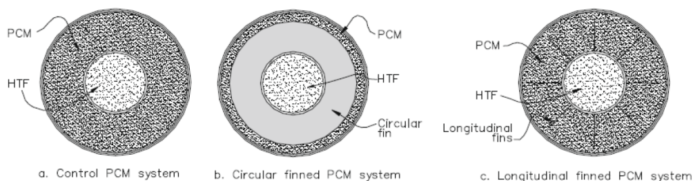
Figure 44 : Les différents types d'échangeurs avec ailettes [83].
