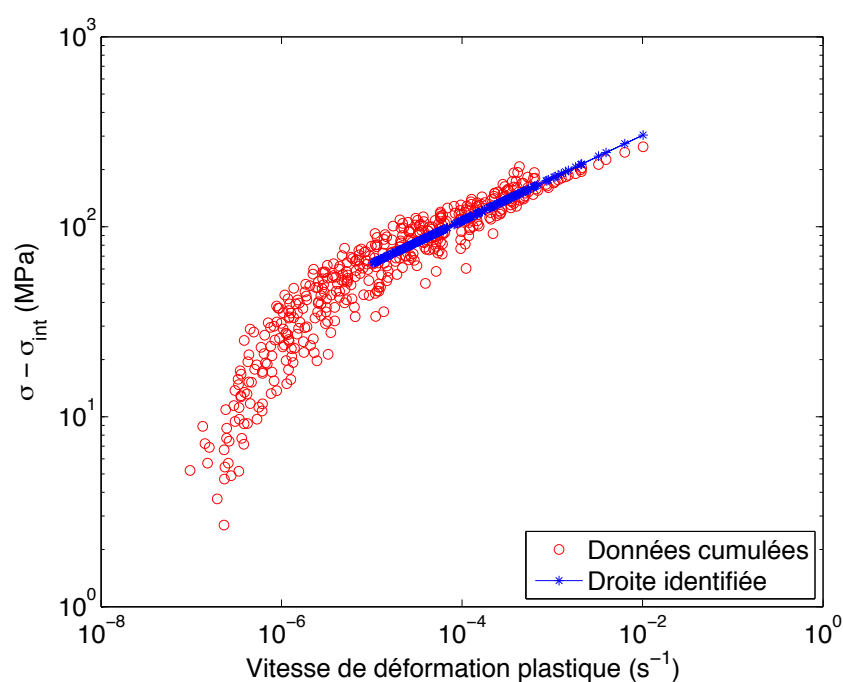
Figure IV - 3 : Identification des paramètres K et n pour les essais de relaxation à 1000^\circ\text{C} (données cumulées des tous les essais réalisés à 1000^\circ\text{C} )
