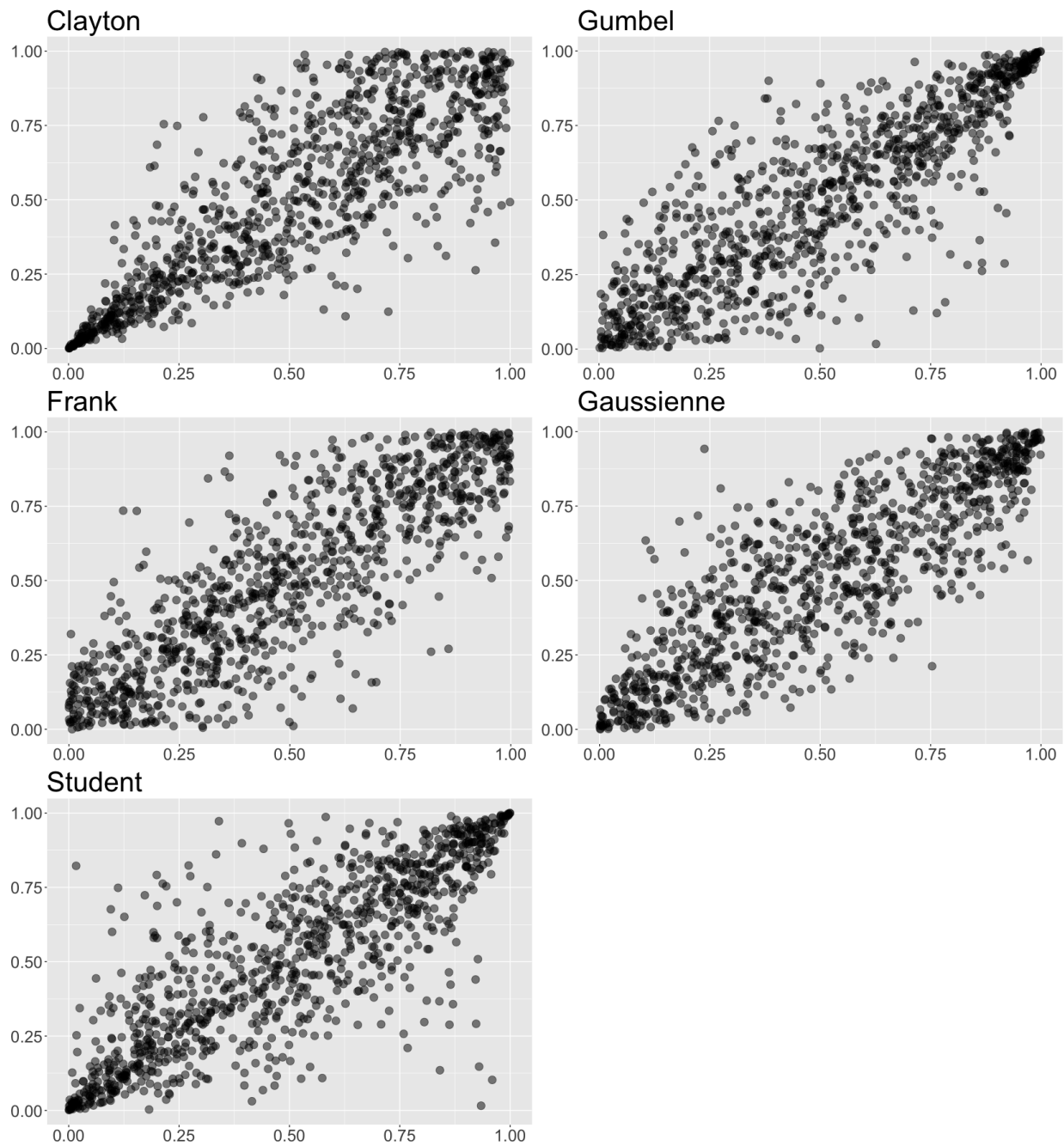
Fig. 1.3: Nuages de points correspondant aux cinq familles de copules présentées à la Section 1.3.2. Le tau de Kendall est fixé à 0.65. Pour la copule de Student, le paramètre donnant le nombre de degrés de liberté est fixé à 3.
