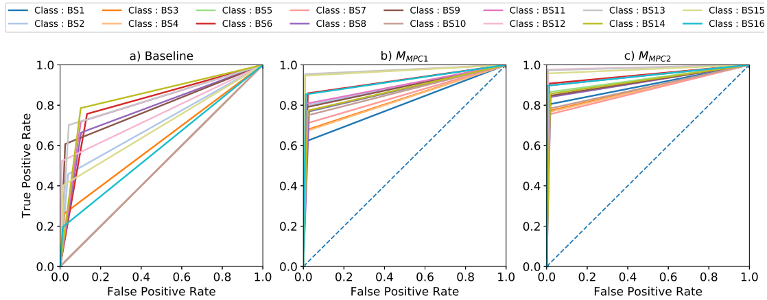
FIGURE 4.16: Performance du modèle MPC (métriques ROC )
