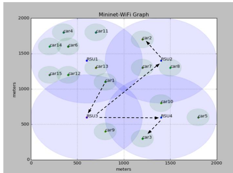
FIGURE 1.12: Scénario de simulation du cas d'utilisation - Phase 2
