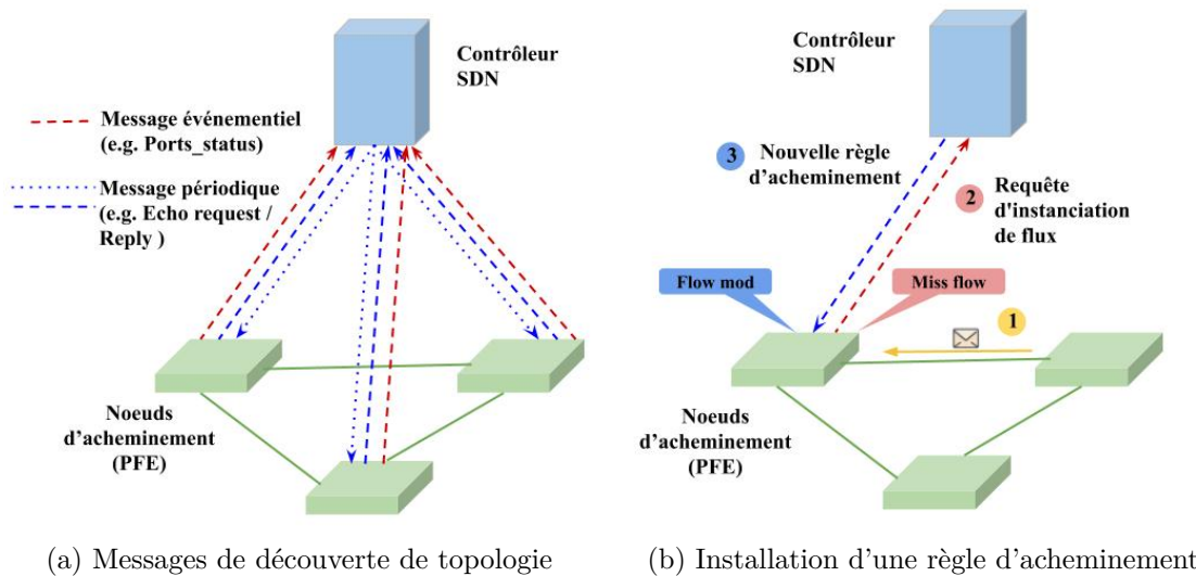
FIGURE 2.1: Exemples d’échanges entre contrôleur et nœuds d’acheminement
