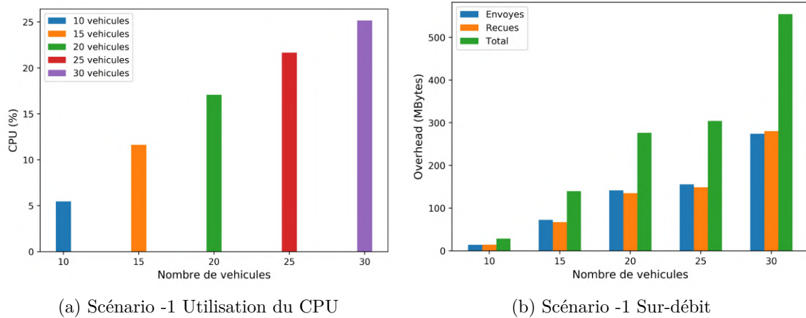
FIGURE 3.6: Scénario -1. Ressources de calcul utilisées et trafic généré par le mécanisme OpenFlow/OFDP
