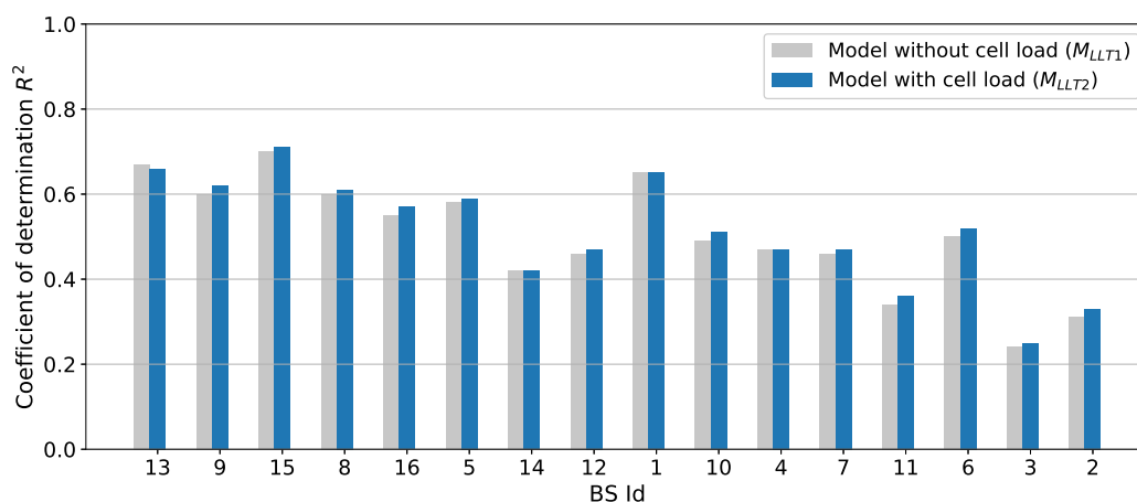
FIGURE 4.12: Performance du modèle LLT ( R^2 )
