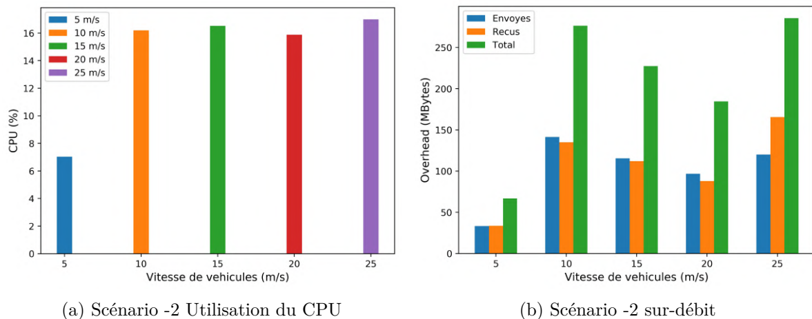
FIGURE 3.7: Scénario -2. Ressources de calcul utilisées et trafic généré par le mécanisme OFDP
