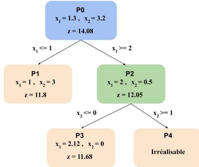
FIGURE 2.10: Arbre de décision construit par la méthode Branch and Bound
