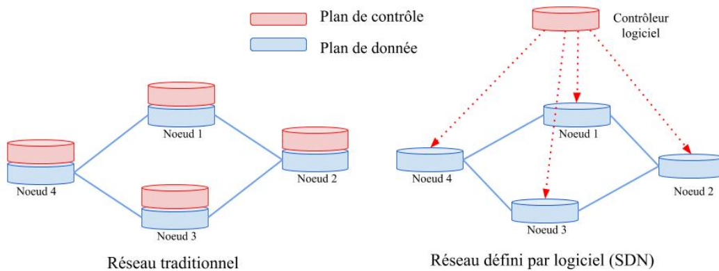
FIGURE 1.4: Réseau traditionnel et réseau défini par logiciel SDN
