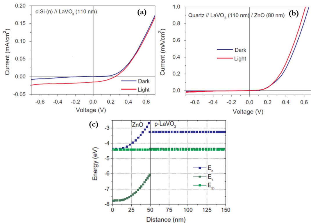
Figure 26 : La caractéristique J-V avec et sans éclairciment du (a) LVO/ZnO et (b) LVO/c-Si. (c) La structure de bande théorique illustrant le décalage de la bande de conduction du ZnO et LVO, adaptée de [32].
