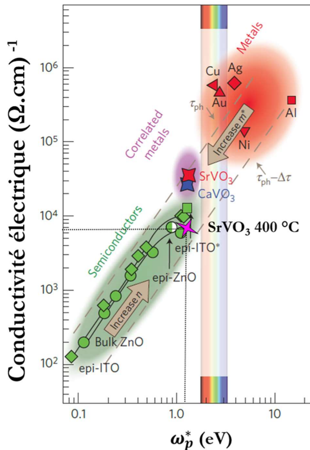
Figure 11 : La figure rassemble la conductivité électrique \sigma et la fréquence plasma écrantée \omega_p^* des métaux corrélés \text{SrVO}_3 (étoile rouge) et \text{CaVO}_3 (étoile bleu) localisés entre les semi-conducteurs dopés (zone verte) et les métaux conventionnels (zone rouge). Notre \text{SrVO}_3 synthétisé à 400 °C (étoile rose) possède une conductivité comparable à celle de l'ITO et une fréquence plasma située en dehors du domaine visible est comparable à celles du \text{SrVO}_3 et \text{CaVO}_3 (adapté de [2]).
