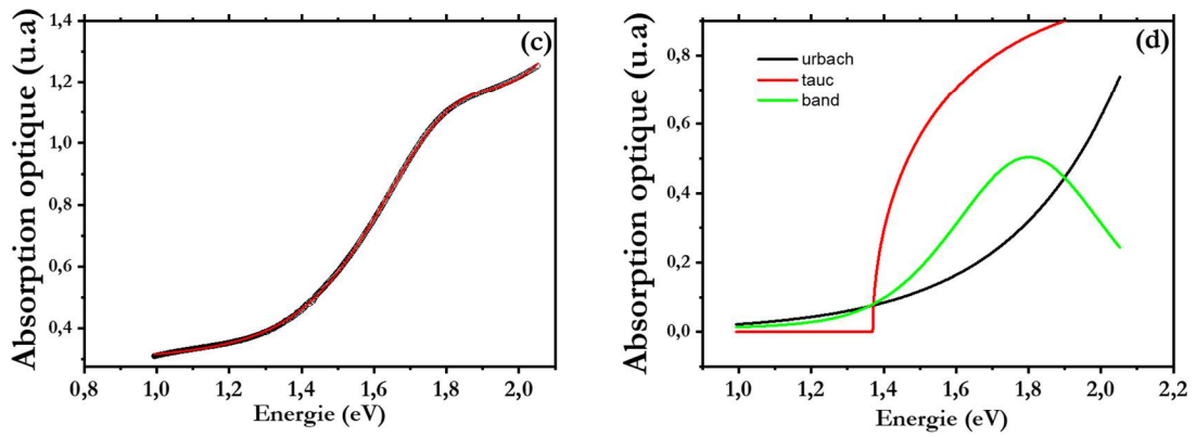
Figure 4 : Ajustement de l'absorption optique du LVO/LSAT 600 °C et 10 -6 mbar et 600°C-10 -5 mbar pour des transition directe permise ( n= \frac{1}{2} ) à l'aide du modèle Exciton, Tauc et Urbach (TEU).
