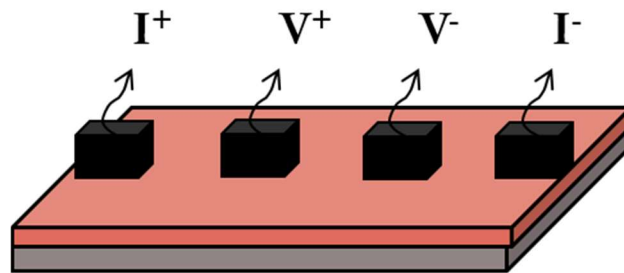
Figure 12 : Mesure de la résistance électrique d'un échantillon en configuration 4 pointes.
