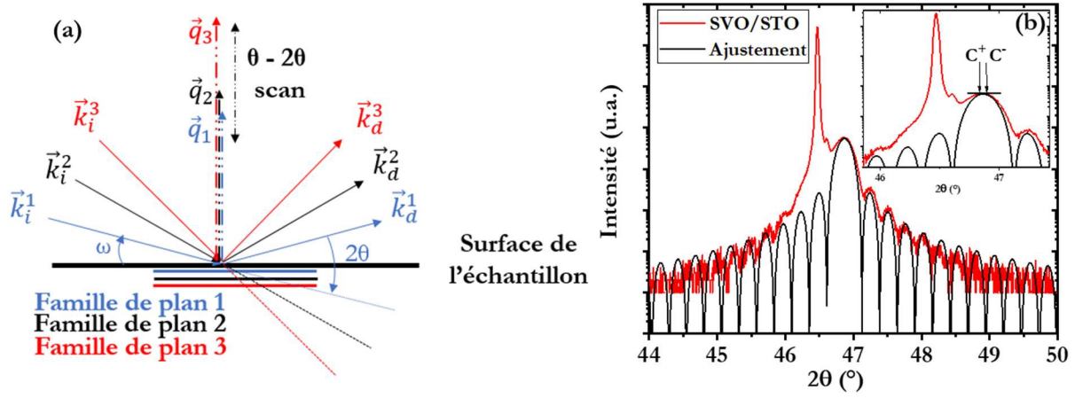
Figure 7 : (a) Représentation graphique d'un \theta-2\theta scan pour différentes familles de plans parallèles à la surface de l'échantillon. (b) Exemple d'une réflexion symétrique effectuée sur un film mince de \text{SrVO}_3 synthétisé sur un substrat \text{SrTiO}_3 ainsi que l'ajustement mathématique des oscillations de Laue.
