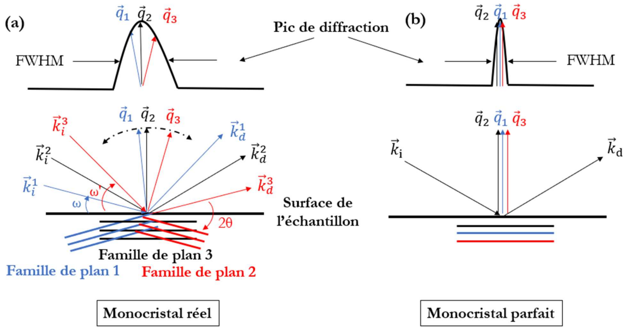
Figure 6 : Représentation graphique d'un \omega -scan pour différentes familles de plans cristallins dans (a) un monocrystal réel et (b) un monocrystal parfait.
