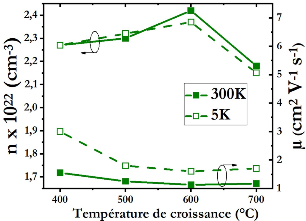
Figure 6 : Dépendance en température de croissance T_G de la densité et la mobilité des porteurs de charges mobiles à 5 et 300 K.
