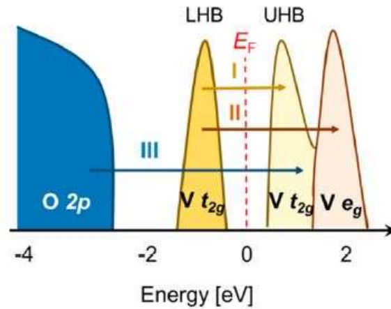
Figure 1 : Structure électronique du \text{LaVO}_3 illustrant les différentes transitions optiques entre les bandes de Hubbard et entre l'orbital 3d du Vanadium et 2p de l'oxygène [31].
