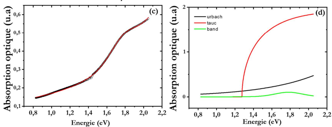
Figure 3 : (a), (c) Ajustement de l'absorption optique du LVO/STO 600 °C et 10 -6 mbar et 600°C-10 -5 mbar pour des transitions directes permises ( n= \frac{1}{2} ). (b), (d) figures récapitulatifs des trois modèles : Urbach (noir), Tauc (rouge) et Exciton (vert).
