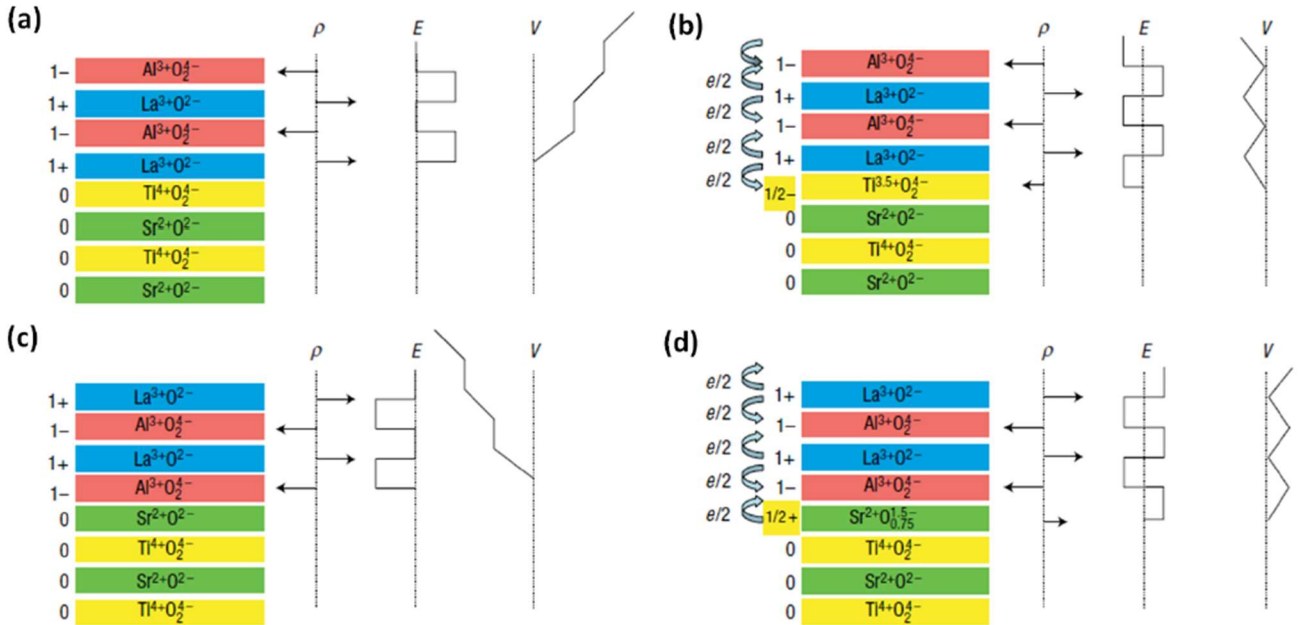
Figure 8 : (a) et (c) Illustration graphique de l'interface (\text{AlO}_2)^- / (\text{LaO})^+ / (\text{TiO}_2)^0 / (\text{SrO})^0 et (\text{LaO})^+ / (\text{AlO}_2)^- / (\text{SrO})^0 / (\text{TiO}_2)^0 qui génèrent un potentiel V divergeant. (b) et (d) Transfert électronique à travers l'interface afin d'éviter la discontinuité polaire, adaptée de [34].
