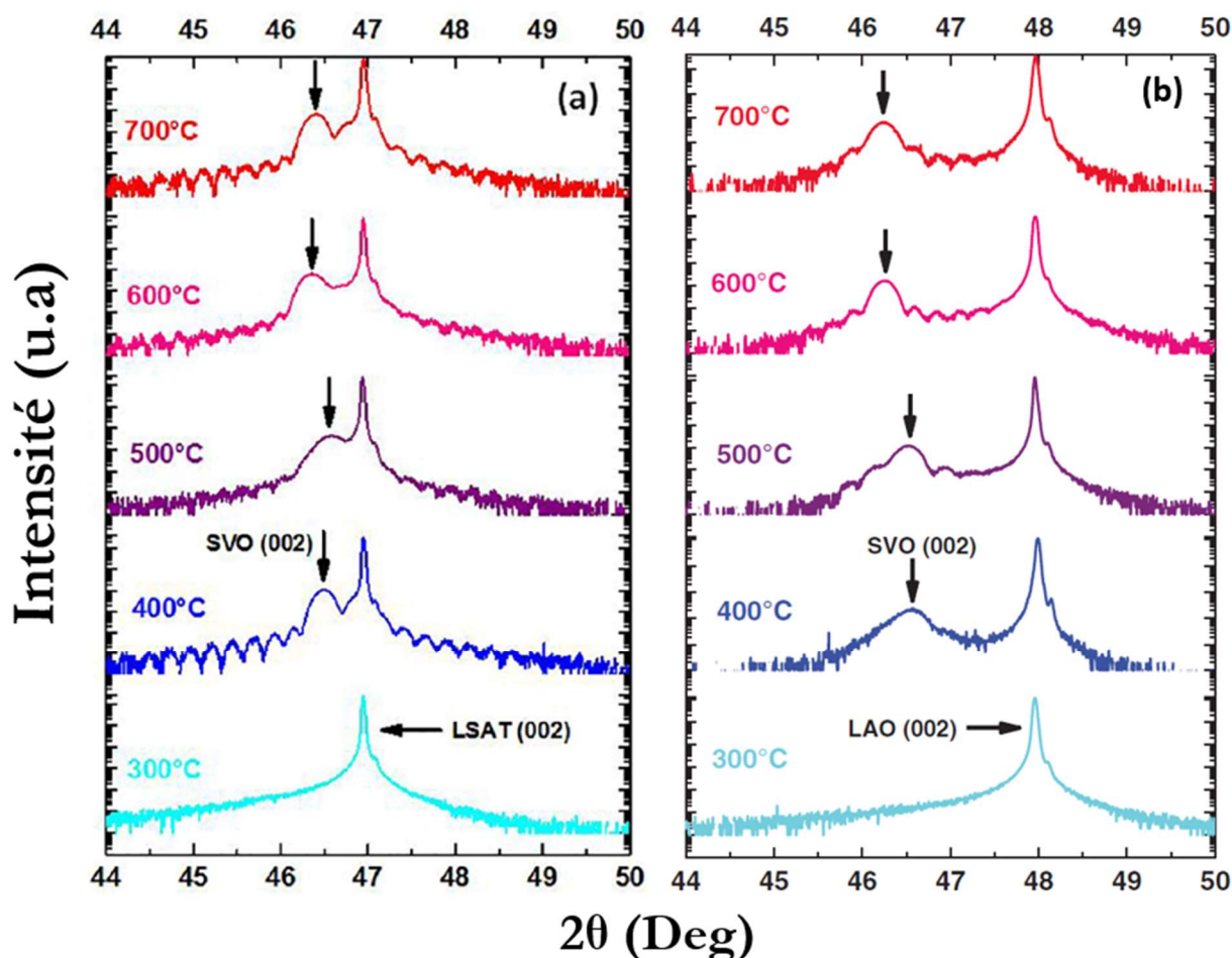
Figure 15 : Diffractogrammes des films \text{SrVO}_3 déposés respectivement sur un substrat de (a) LSAT et (b) \text{LaAlO}_3 entre 300 et 700 °C en configuration Bragg-Brentano autour de la raie symétrique (002) du LSAT et LAO.
