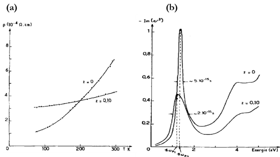
Figure 12 : (a) Dépendance en température de la résistivité du \text{SrVO}_{2,9} et \text{SrVO}_3 , (b) l'évolution en énergie de la fonction perte d'énergie des deux composés, adaptée de [61].
