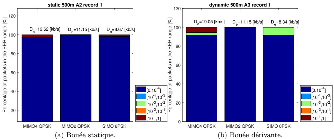
FIGURE I.6 – Performances du récepteur du modem acoustique MIMO en fonction des différents modes considérés [63].
