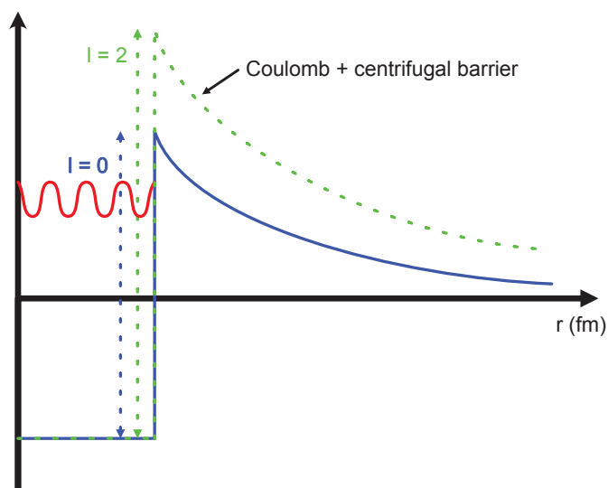
Figure 7.5: Représentation schématique de la barrière coulombienne et centrifuge pour l=0 et l=2 . Dans le noyau les protons et neutrons sont piégés dans ce que l'on appelle un puits de potentiel. L'onde sinusoïdale en rouge représente un nucleon piégé par la barrière coulombienne (et centrifuge pour l>0 ).
