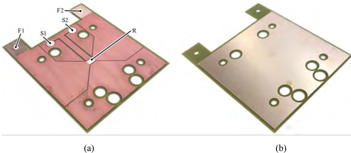
Figure 3.1 – Vue du substrat en face supérieure (a) et inférieure (b)
