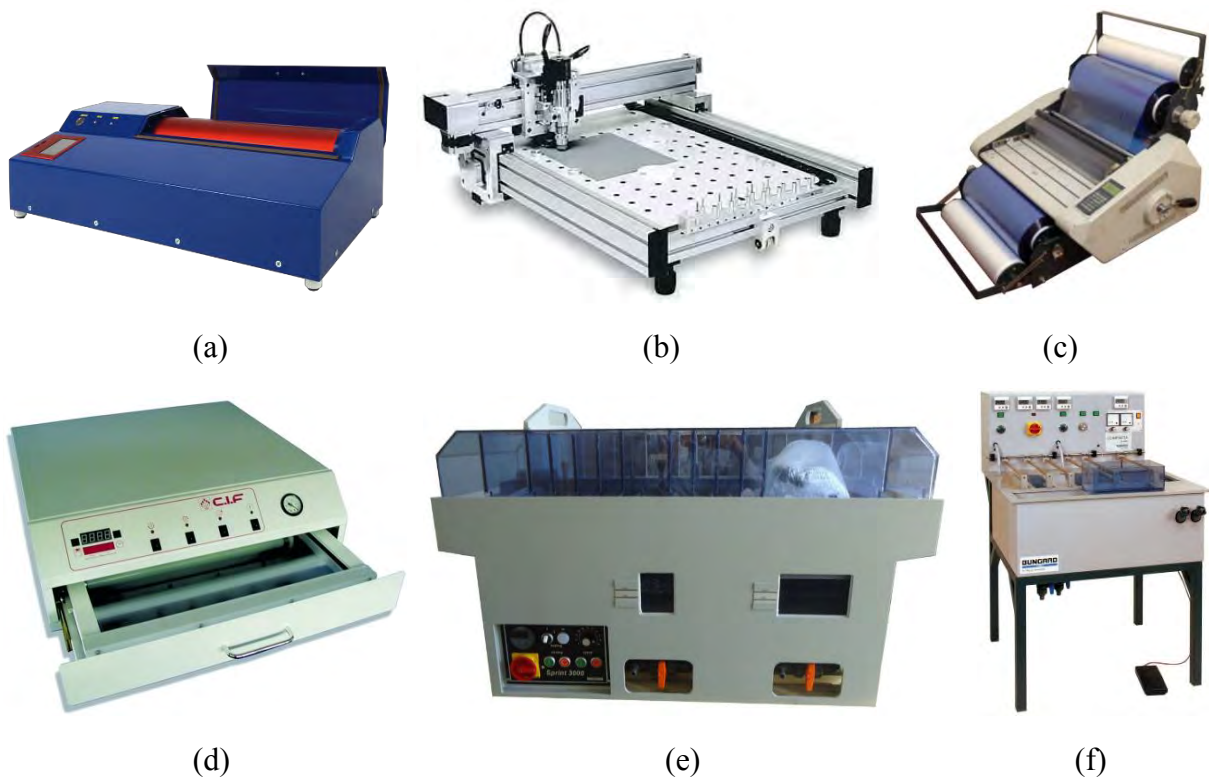
Figure 2.40 – Photoplotter FP 3000 Cypax (a), micro-fraiseuse CCD/ATC Bungard (b), lamineur M300 Eurolam (c), insoleuse DST 3040 CIF (d), graveuse chimique Sprint 3000 Bungard (e) et banc d'électrodéposition Compacta 30 Bungard (f)
