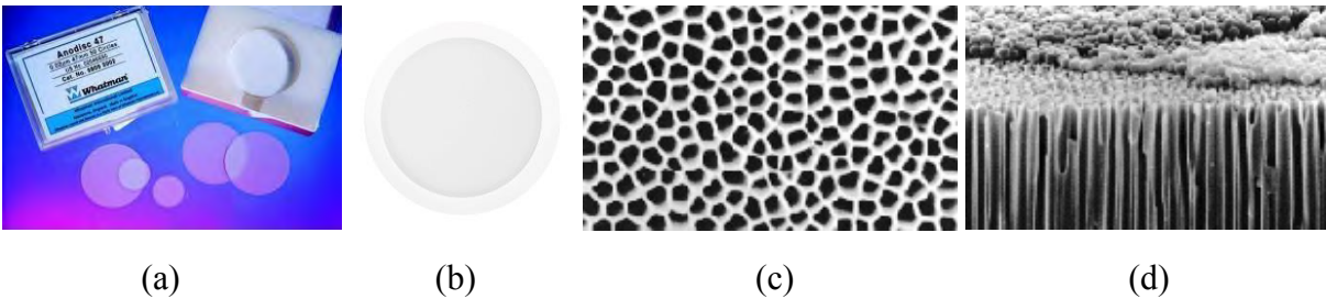
Figure 2.15 - Boîte (a) et membrane (b) Whatman® Anodisc™ 47 avec vue de dessus (c) et de profile (d) (Whatman)
