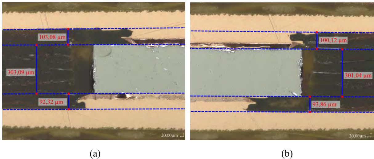
Figure 3.27 – Images au microscope numérique (x300) des extrémités de la puce interconnectée
