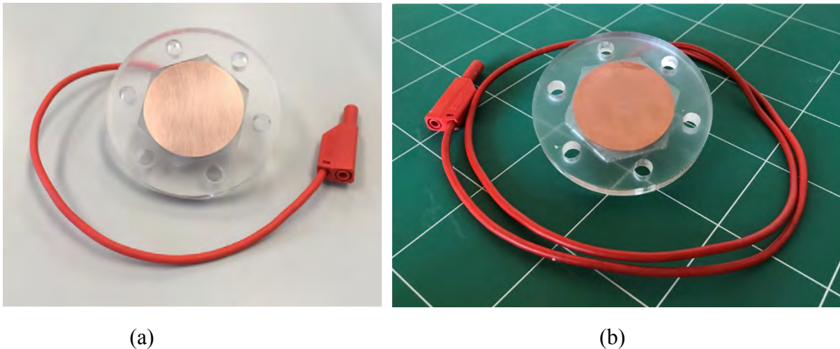
Figure 2.24 – Anode après assemblage avec polissage (a) puis rodage et traitement chimique (b)
