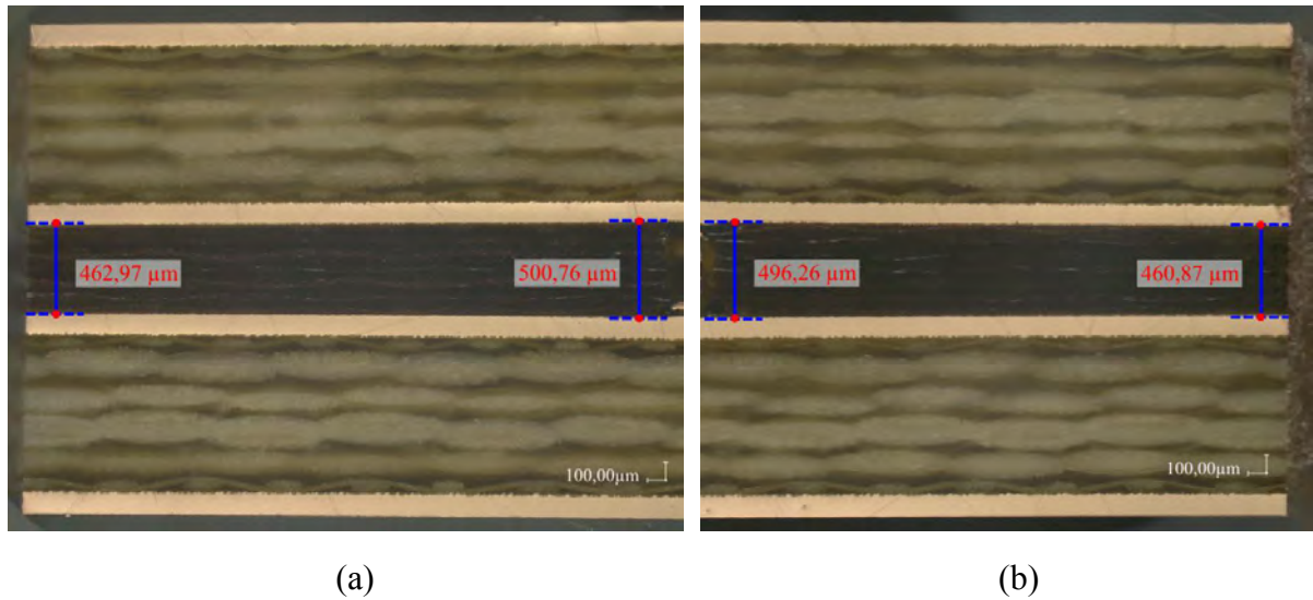
Figure 3.26 – Images au microscope numérique (x100) de la mesure du diélectrique central
