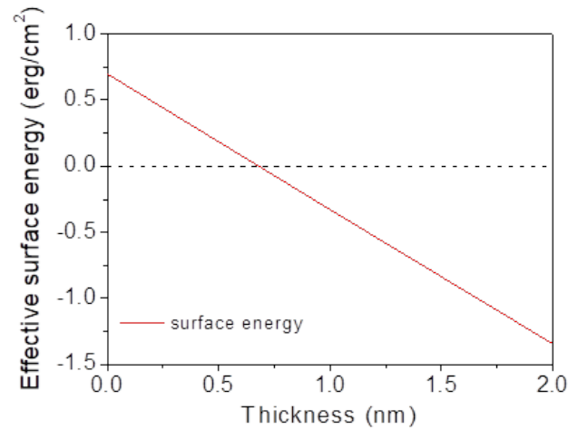
FIGURE A.1 – Simulation de l'énergie de surface effective en fonction de l'épaisseur t de la couche de CoFeB à partir des paramètres suivants : M_s = 1350 emu/cc, K_v = 1,2 Merg/cc et K_s = 0,7 erg/cm 2
