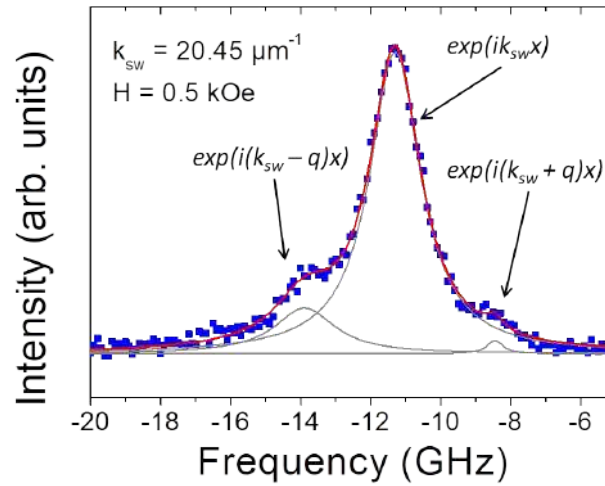
FIGURE 6.16 – Zoom d'un spectre BLS montrant trois raies Stokes distinctes dont la raie principale correspondant au pic le plus intense. Les symboles se réfèrent aux données expérimentales et les lignes continues aux fits Lorentziens.
