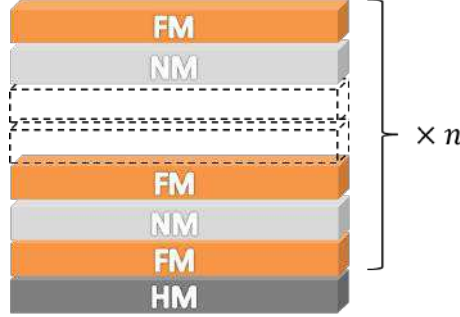
FIGURE 3.11 – Système d'empilement de couche composé de n couches ferromagnétiques (FM) séparées par un espaceur non-magnétique (NM) et déposées sur une seule couche de métal lourd (HM) afin d'induire la DMI.
