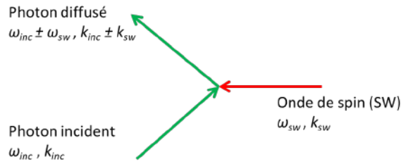
FIGURE 2.5 – Principe de la diffusion Brillouin.
