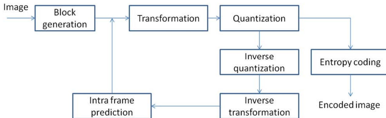
Figure 2.11 : Schéma d'encodage d'un codec "block-based" adopté par le format WebP
