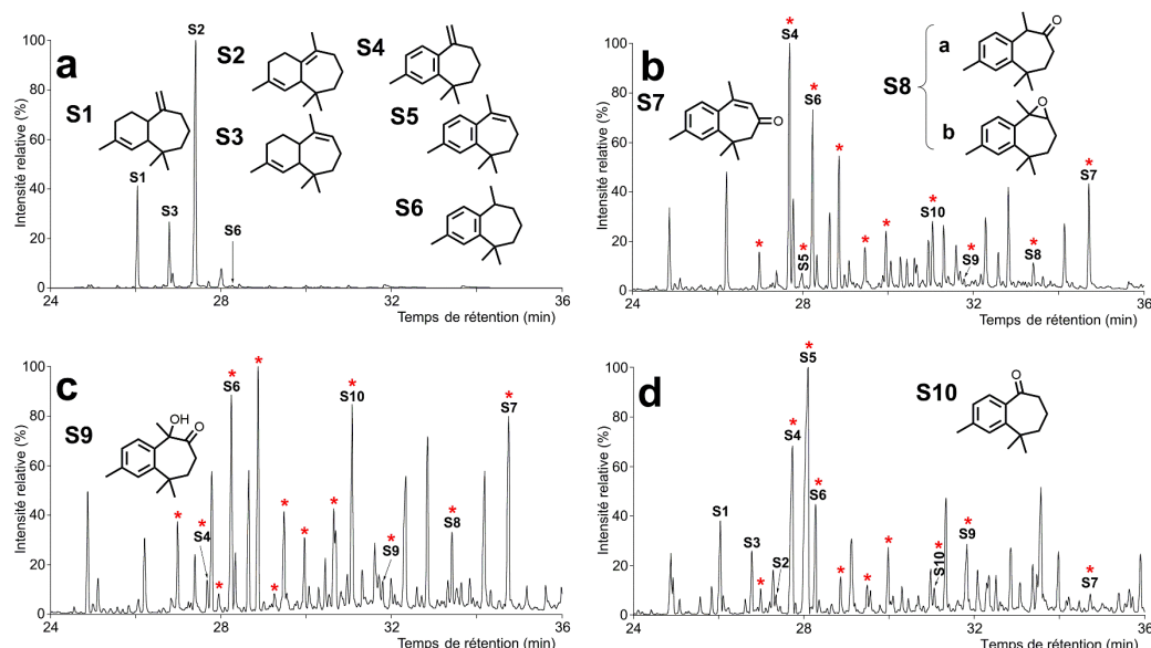
Figure 2.6 : Chromatogrammes en phase gazeuse partiels (GC-MS, IE, 70 eV) de l'huile essentielle de cèdre de l'Atlas avant oxydation (a) ; de l'extrait au pentane après 20 h et 92 h d'oxydation dans CH 3 CN (b, c) ; de l'extrait au pentane après 92 h d'oxydation dans AcOH (d). Les étoiles rouges indiquent les composés également mis en évidence dans des vases égyptiens (Sarret et al., (2017). Les structures des composés numérotés sont représentées dans l'Appendice de la thèse. Programme A de température du four GC (cf. § 6.5.2).
