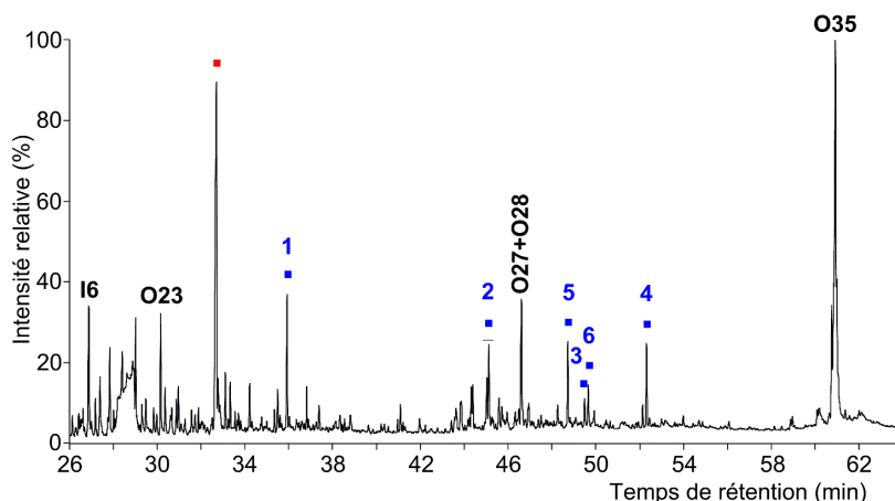
Figure 2.28 : Chromatogramme en phase gazeuse partiel (GC-MS, IE, 70 eV) de l'extrait lipidique obtenu après oxydation pendant 20 h d'un mélange d'huile essentielle de baies de genévrier et de linoléate de méthyle I5 . Le carré rouge indique la présence d'un composé azoté dérivé du NHPI. Les carrés bleus numérotés de 1 à 6 correspondent à de nouveaux composés mis en évidence par rapport à l'altération par autoxydation du linoléate de méthyle I5 seul. Les alcools sont analysés sous forme d'éthers de triméthylsilyle et les acides sous forme d'esters méthyliques. Les structures des composés numérotés sont représentées dans l'Appendice de la thèse. Programme A de température du four GC (cf. § 6.5.2).
