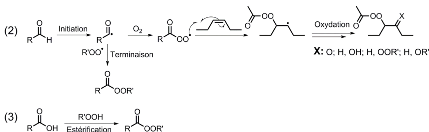
Figure 2.34 : Voies proposées pour la formation des ponts peroxydes et peresters à l'origine de l'oligomérisation de la résine lors de l'autoxydation
